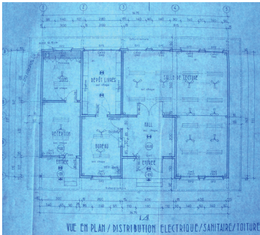
標準設計 図書室棟
