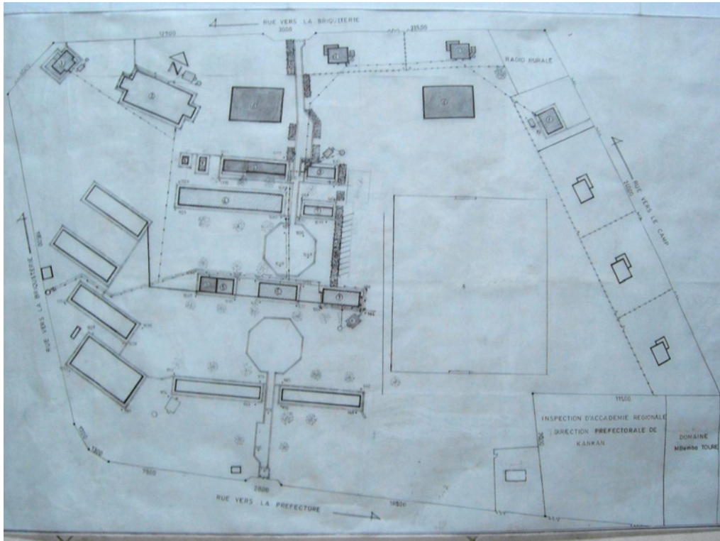
カンカン小学校教員養成校 配置図
