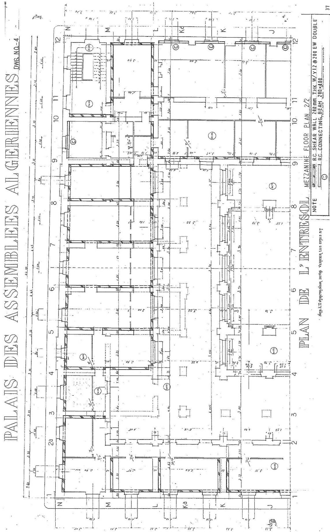
Figure 10-13 Plan de renforcement de l'entresol (2/2)
