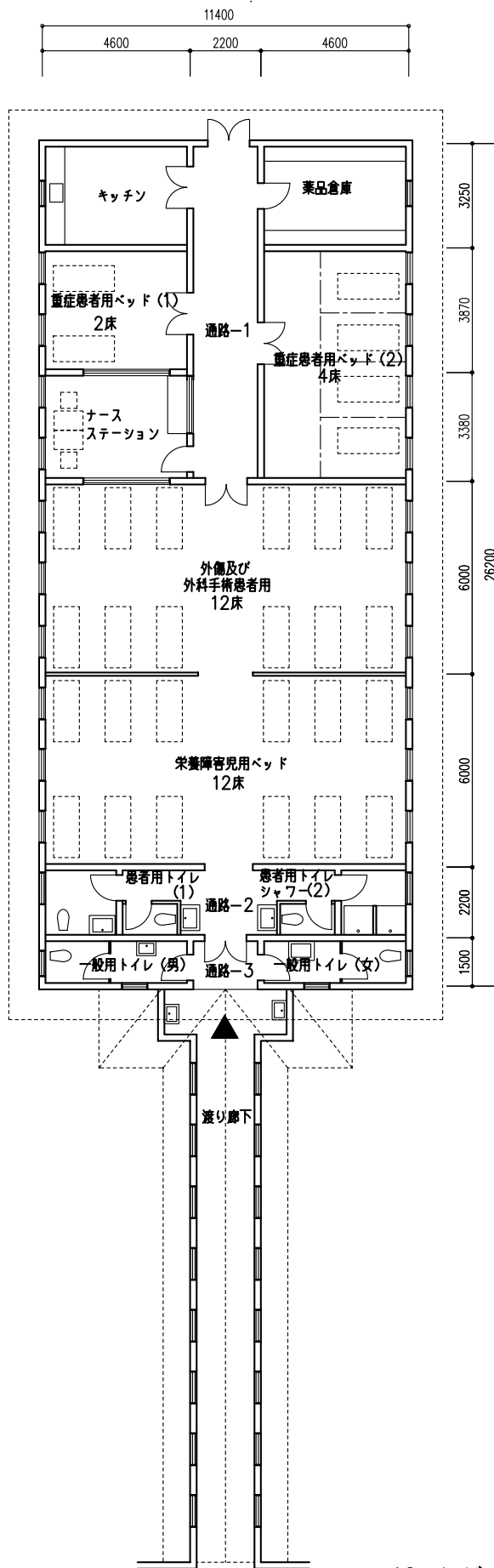
13. ムジンバ県病院 小児科病棟平面図 マラウィ国地方保健医療施設改善計画基本設計調査
