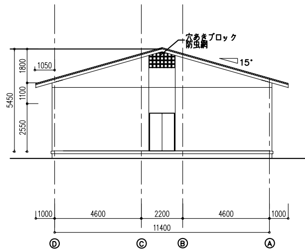
東側立面図
