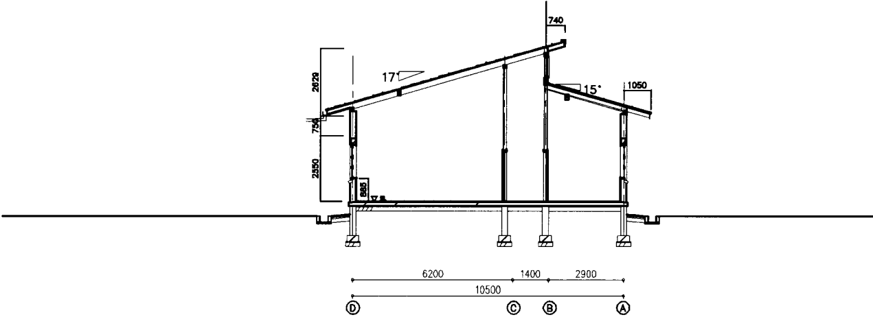
産科棟断面図
