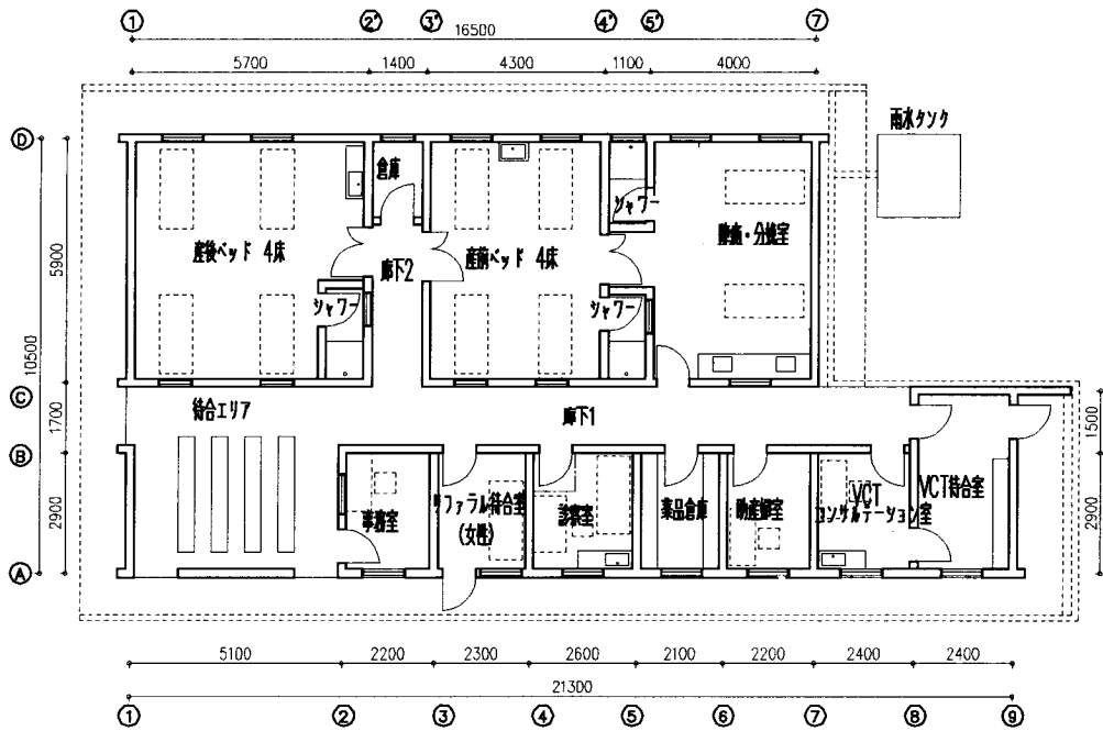
産科棟平面図
