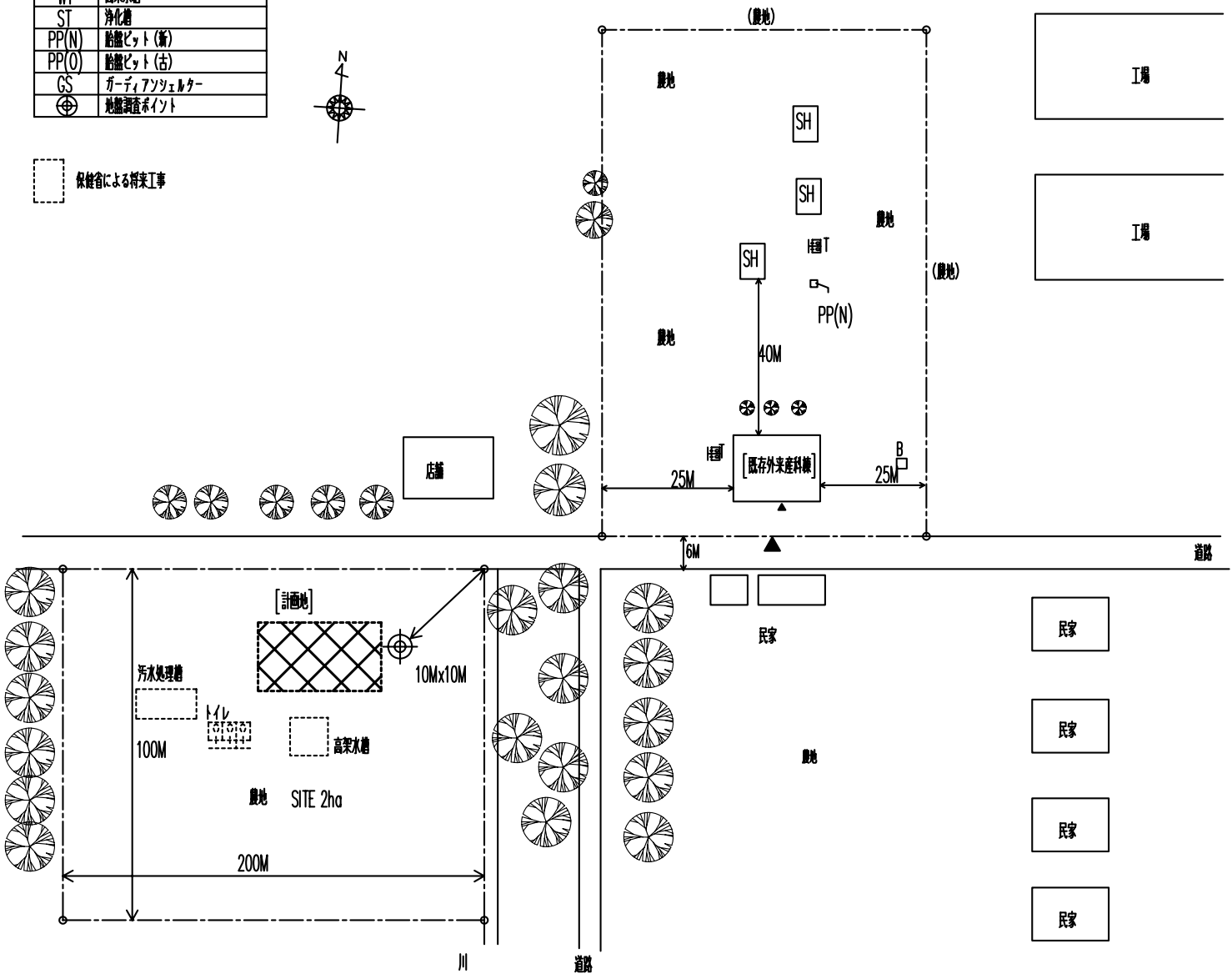
配置図
