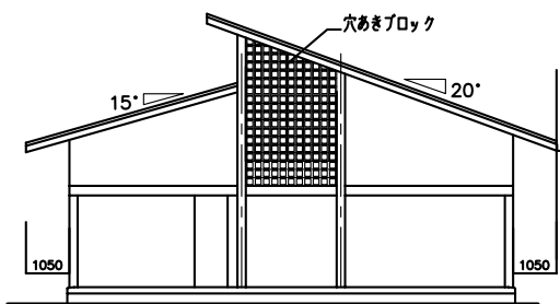
外来棟立面図-3
