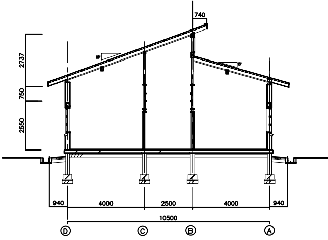
外来棟断面図
