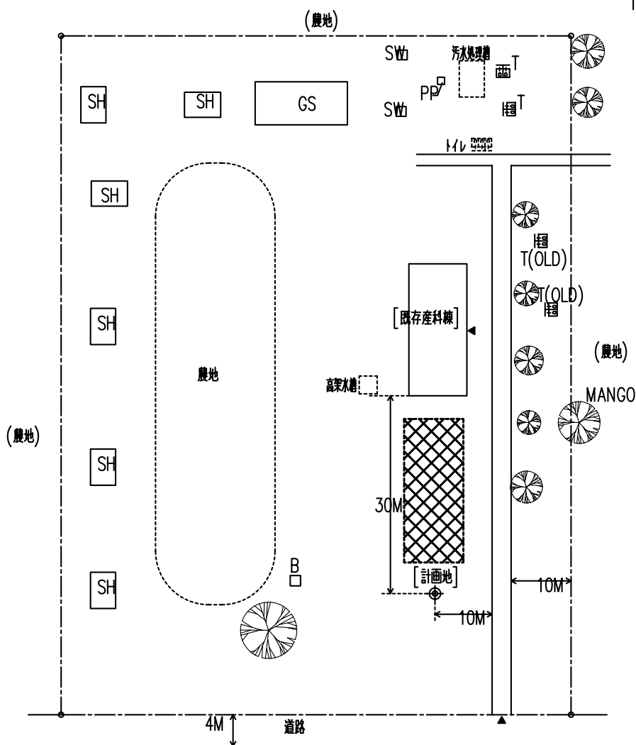
配置図
