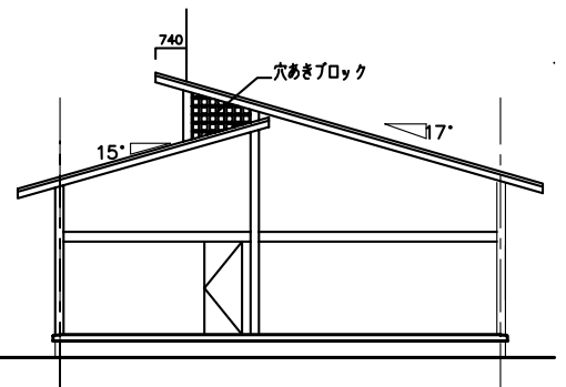
産科棟立面図-4
