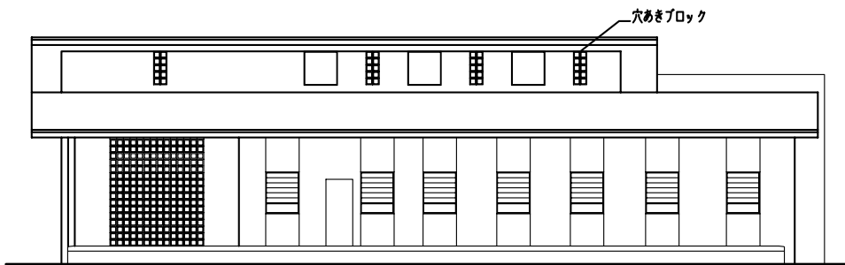
産科棟立面図-1
