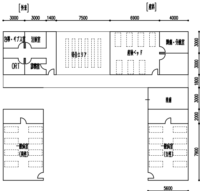
既存平面図
