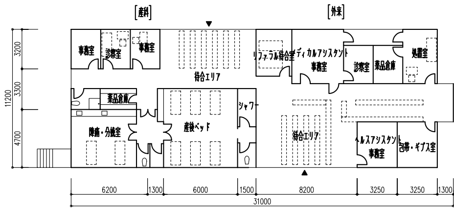
0 5M 既存平面図
