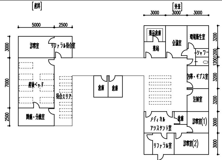
24. LHC-1 チワムバ・ヘルスセンター 外来棟 マラウィ国地方保健医療施設改善計画基本設計調査
