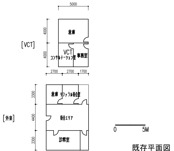
18. MHC-12 カフクレ・ヘルスセンター 外来棟 マラウィ国地方保健医療施設改善計画基本設計調査
