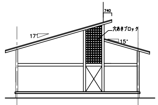
産科棟立面図-2
