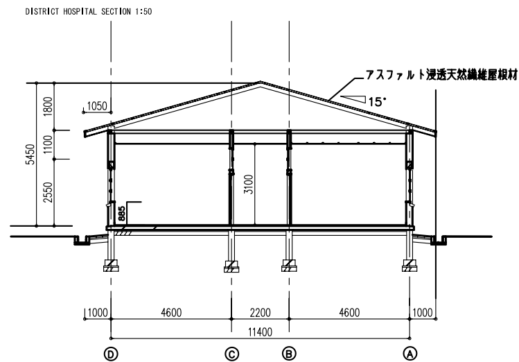
断面図
