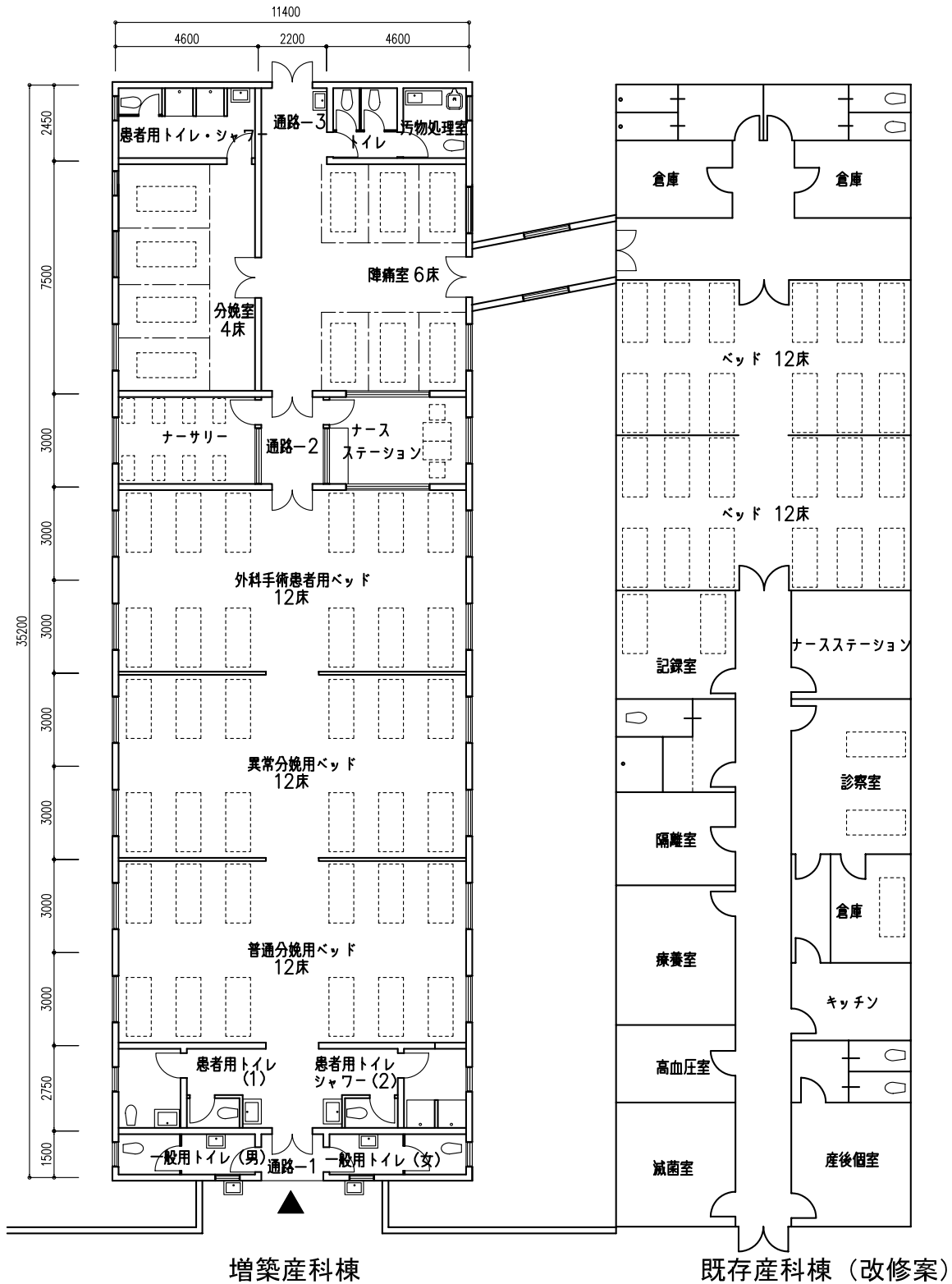
8. ルンピ県病院 産科病棟平面図 マラウイ国地方保健医療施設改善計画基本設計調査
