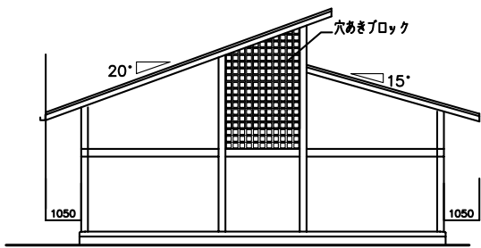
外来棟立面図-1
