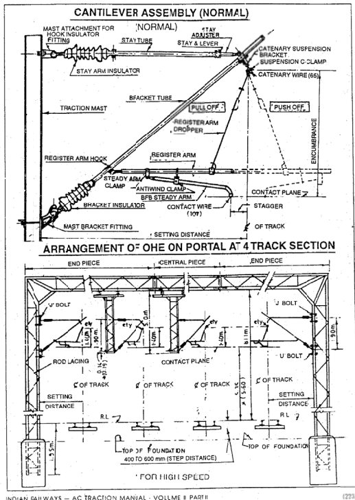
別添資料 図 7-46 電車線路設備技術図
