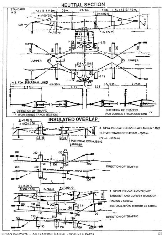
別添資料 図 7-48 電車線路設備技術図
