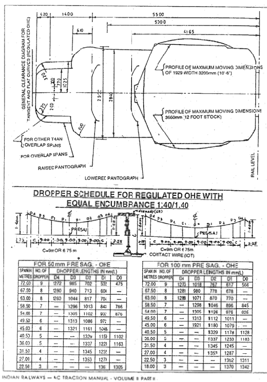
別添資料 図 7- 42 電車線路設備技術図
