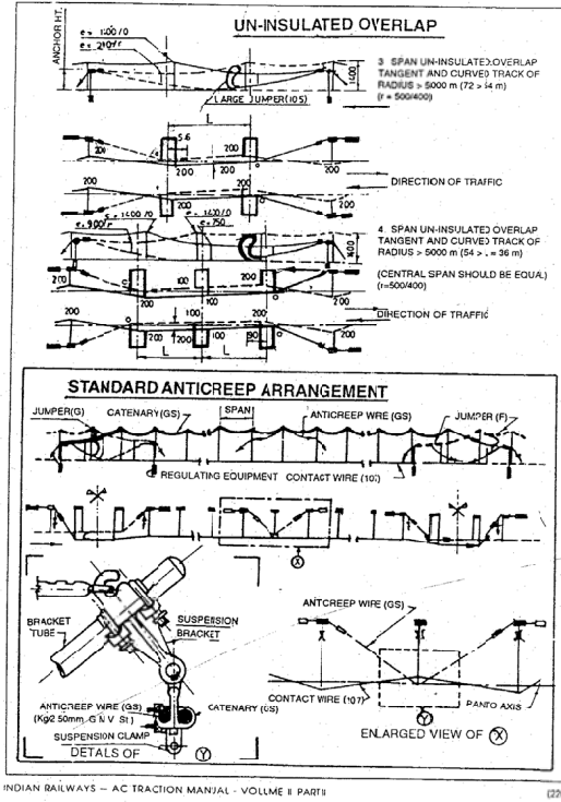
別添資料 図 7-47 電車線路設備技術図
