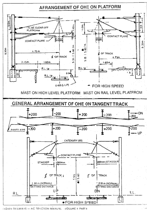
別添資料 図 7- 45 電車線路設備技術図
