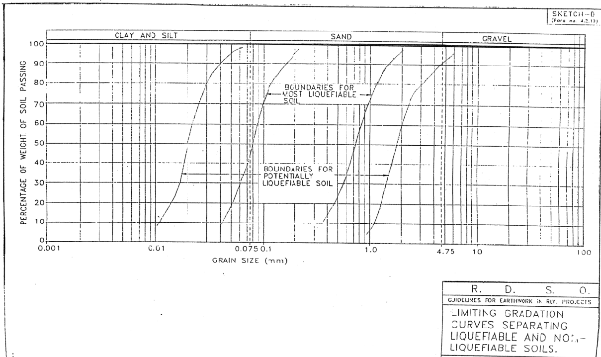
別添資料 図 7- 11 インド国鉄の土工定規 複線区間の盛り土の特性カーブ
