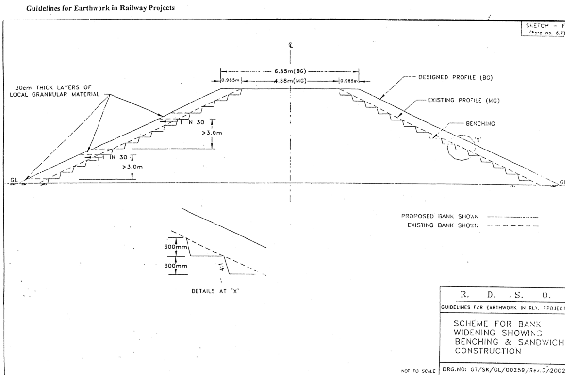
別添資料 図 7- 13 インド国鉄の土工定規
