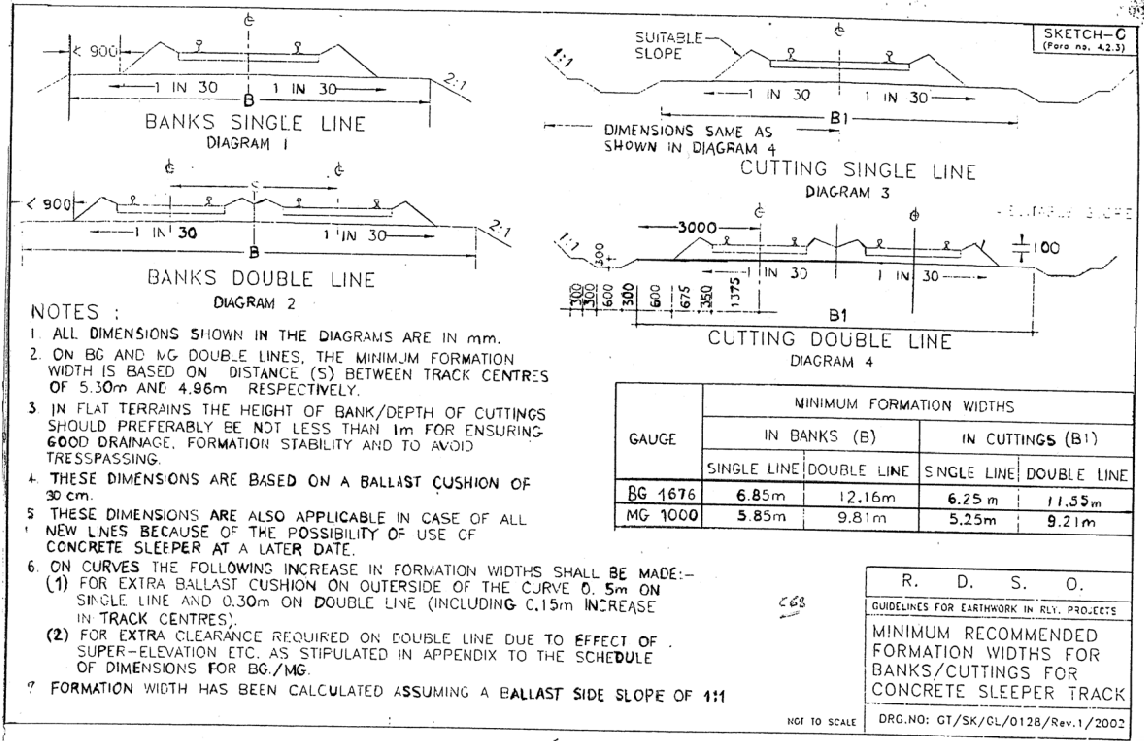
別添資料 図 7- 10 インド国鉄の土工定規 複線区間
