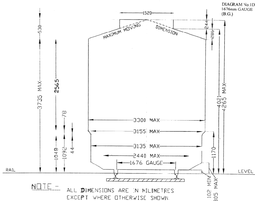
別添資料 図7-5 インドの車両限界図 改定提案図(非電化用)
