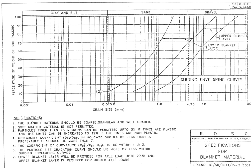
別添資料 図7-9 インド国鉄の土工定規 単線区間の盛り土の特性カーブ
