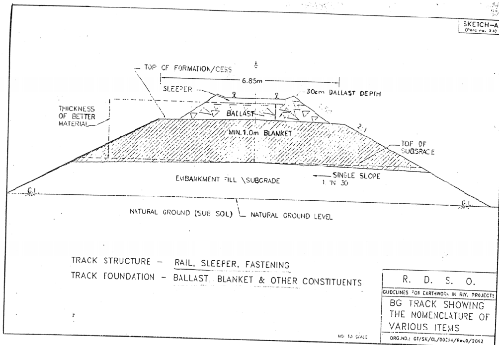
別添資料 図7-8 インド国鉄の土工定規 単線区間
