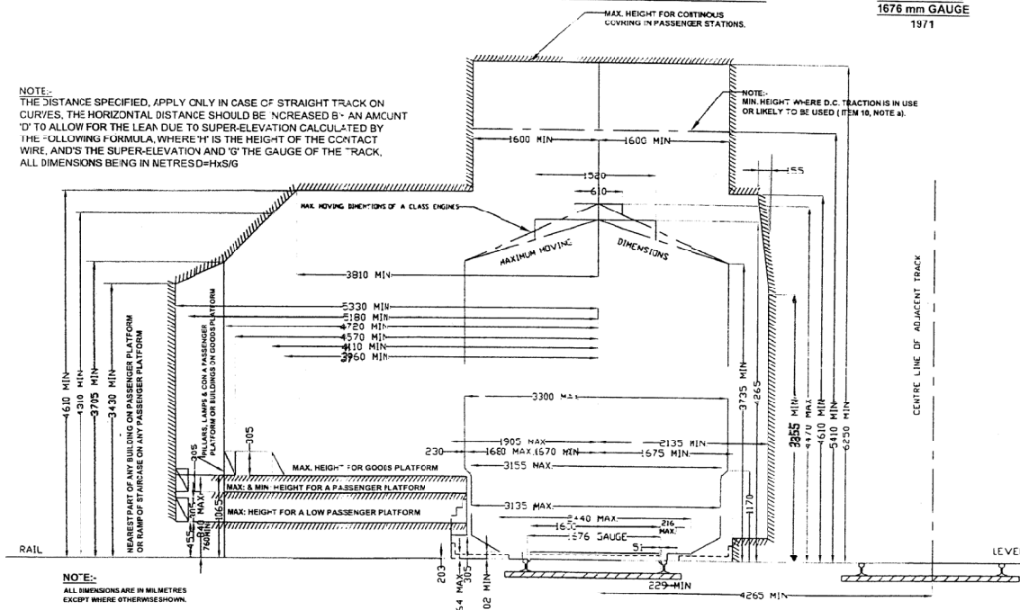
別添資料 図7-6 インドの建設限界と車両限界 25KV AC 電化用(駅用)
