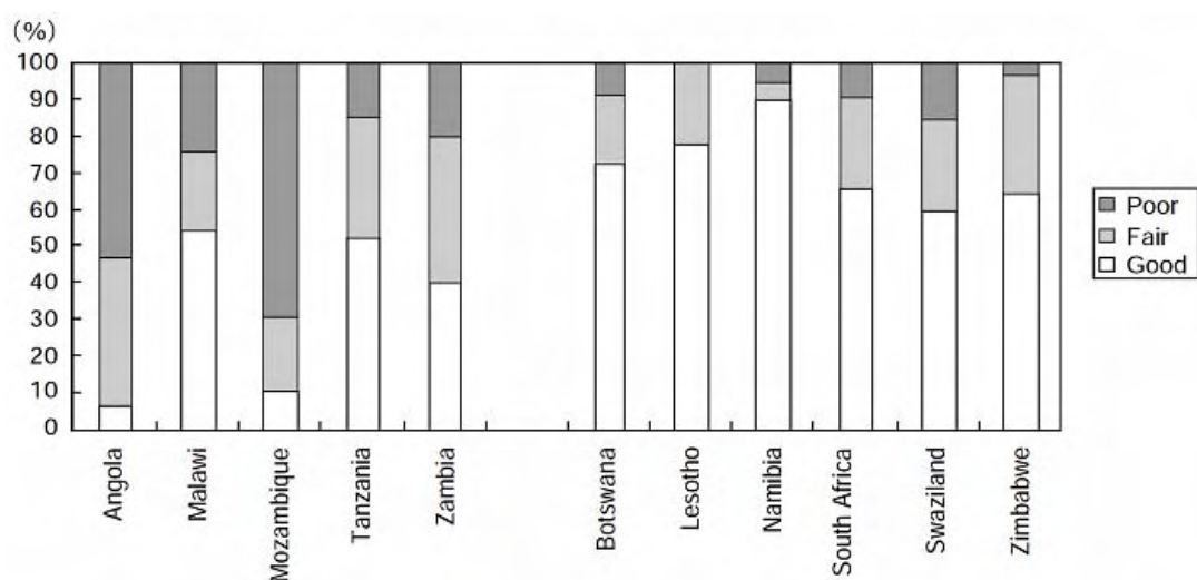
図参考- 18 南部アフリカ開発共同体(SADC)諸国の主要舗装道路の整備水準
