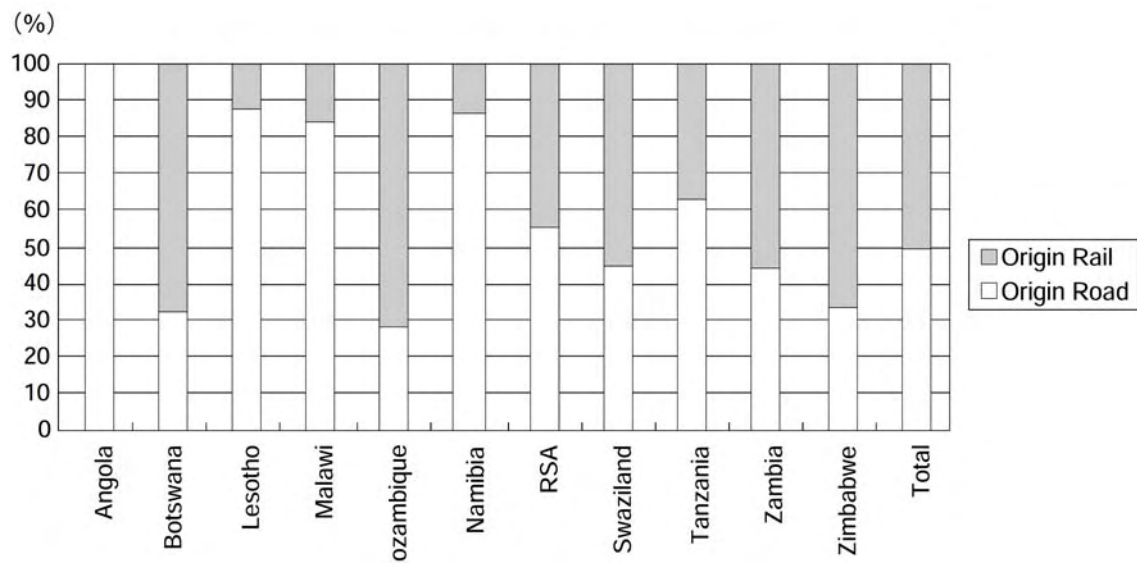
図参考- 28 SADC 諸国発国際貨物の鉄道・道路分担率
