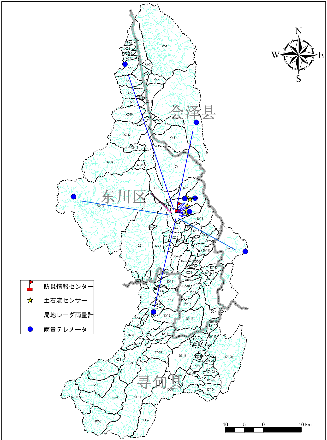
図 I.2 小江流域予警報システムの観測網
