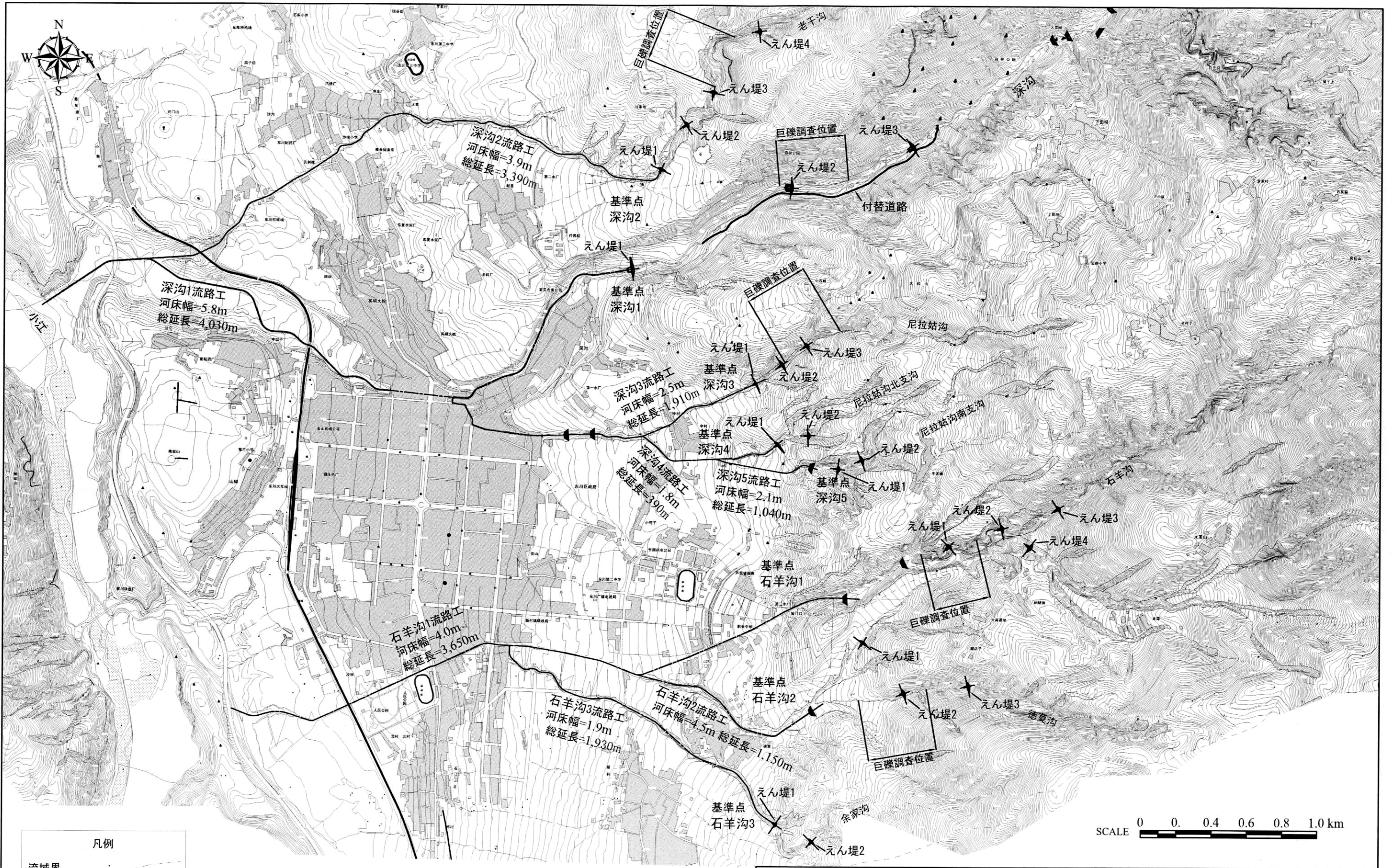
図 G.11 东川区市街地流域土石流構造物対策 配置平面図
