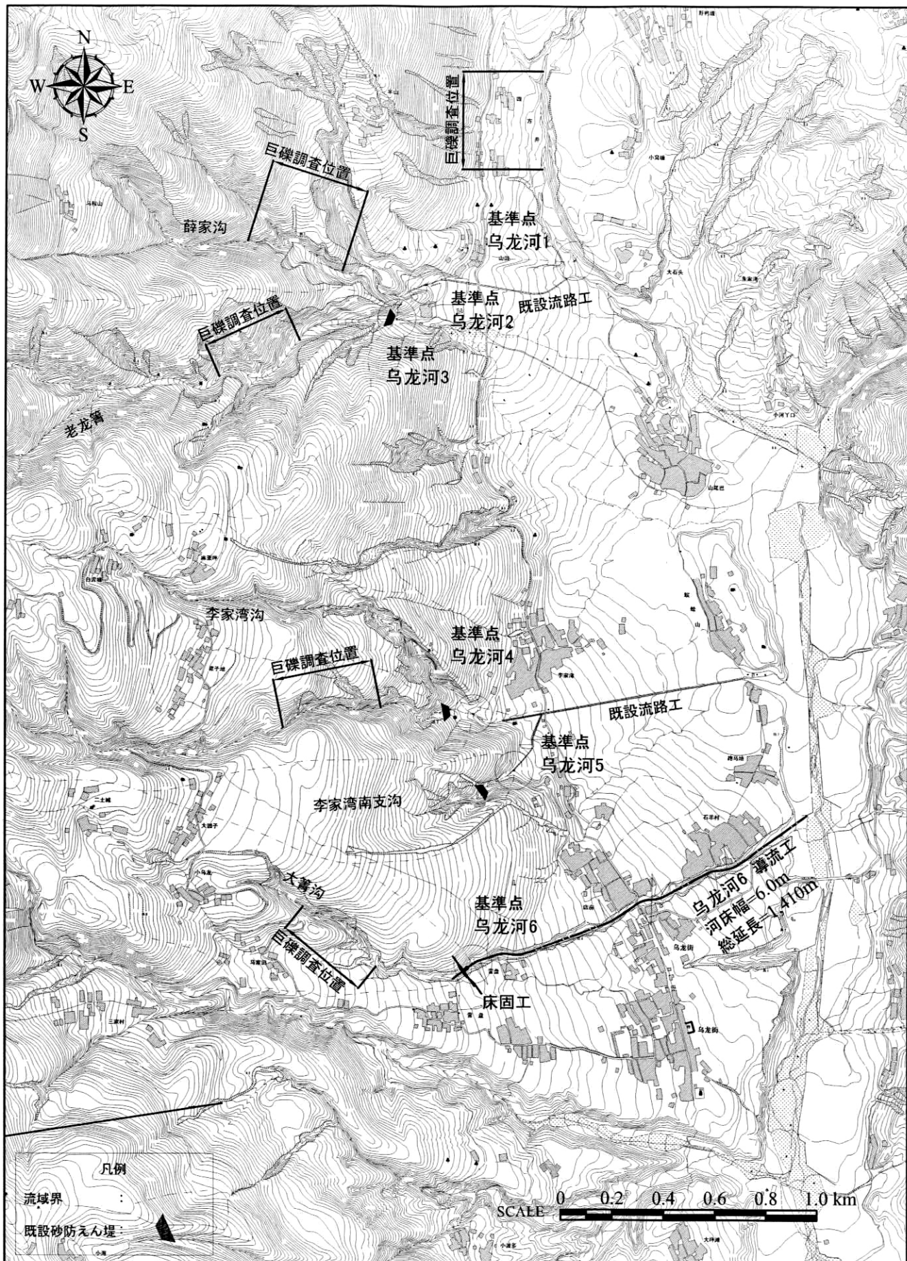
図 G.8 乌龙河流域土石流構造物対策配置平面図
