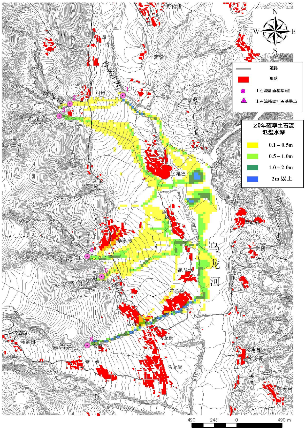
圖 G.7 乌龙河流域土石流氾濫域圖 (20年確率)
