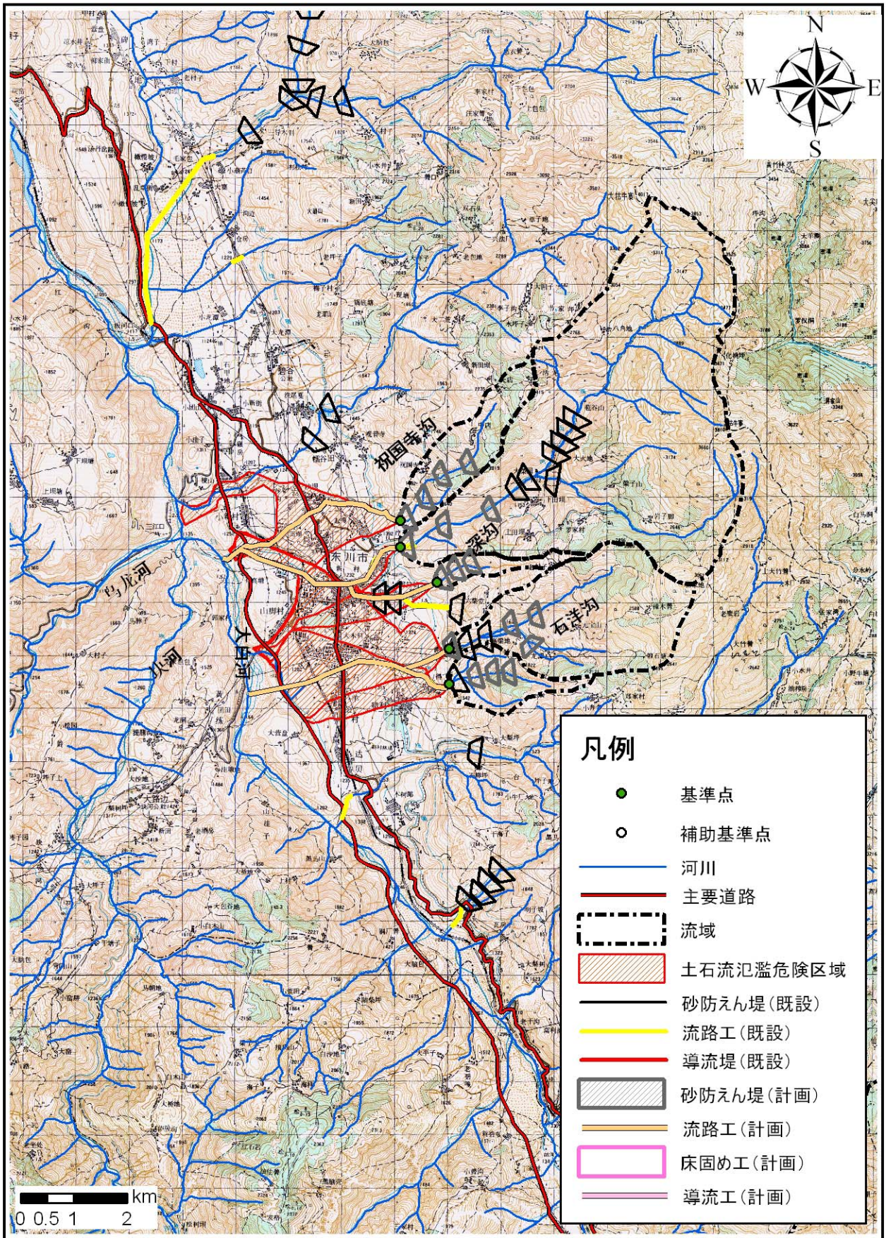
図 G.3(3/4) 土石流対策計画砂防えん堤位置図 (東川市街地域)
