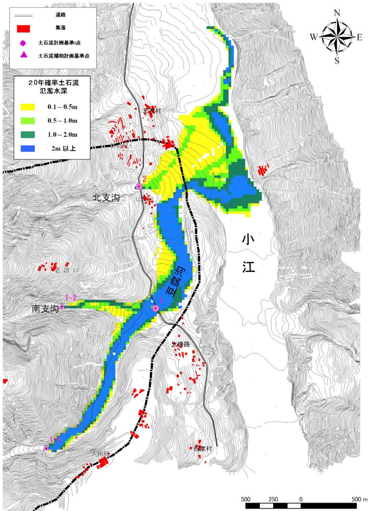
圖 4.2.1 豆腐沟土石流氾濫域圖 (20年確率)
