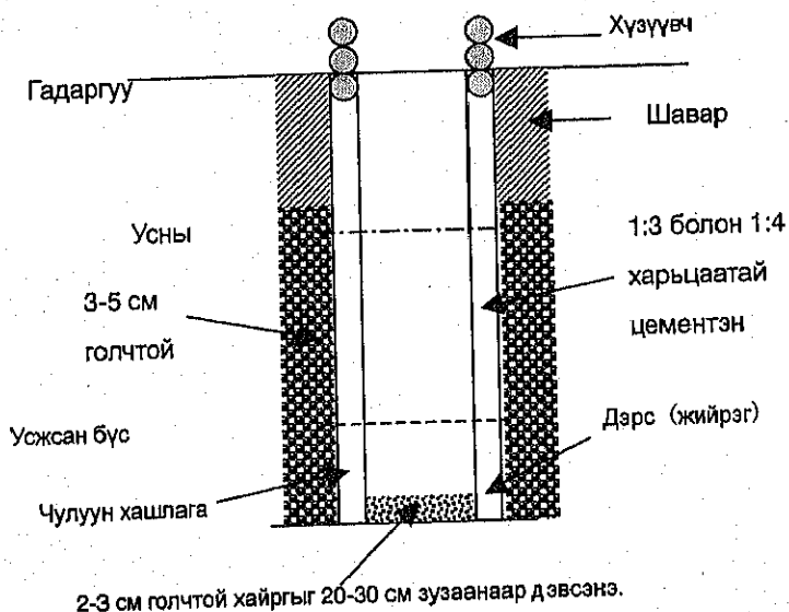
Зураг 4.6.21 Гар худгийн бүтэц
