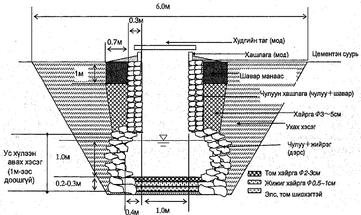
Зураг 4.6.20 Чулуугаар хашсан худгийн бүтэц
