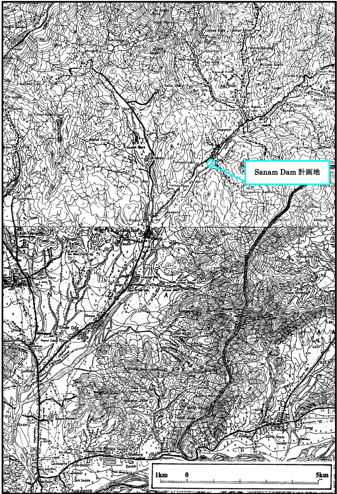
サナムダム計画地および周辺図
