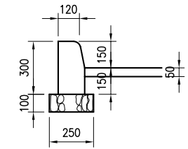
CURB TYPE-A SCALE 1:30
