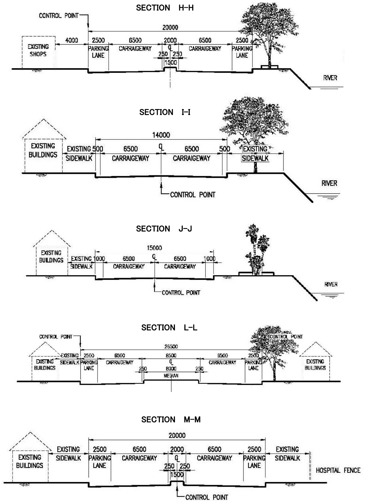
图-5.5.11 標準道路断面图-2
