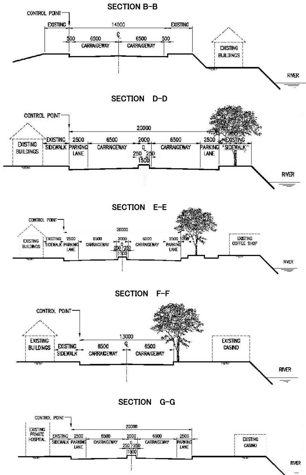
图-5.5.10 標準道路断面图-1
