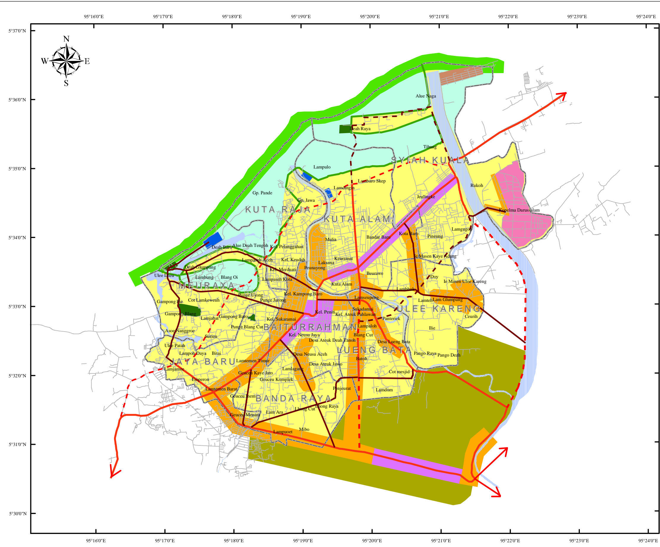
Landuse Plan for Banda Aceh City
