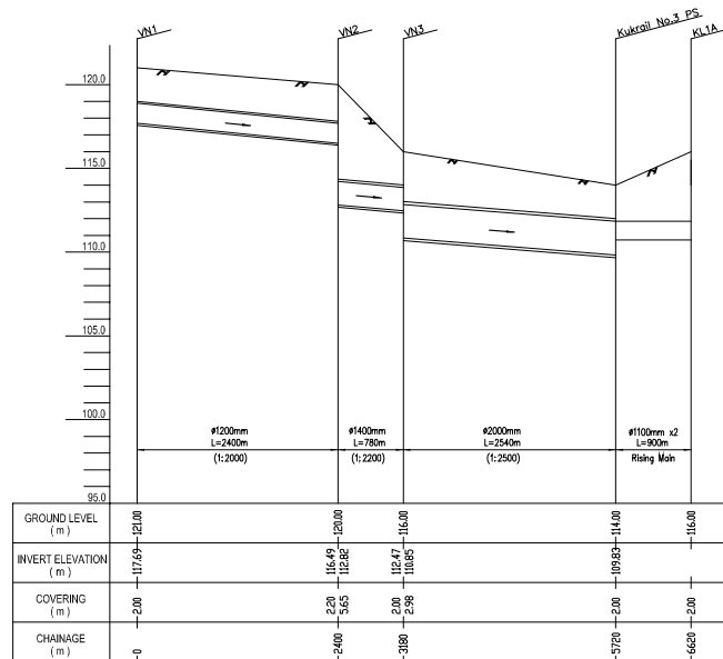
1h PROFILE VIKAS NAGAR SEWER (VN1-KL1A)
