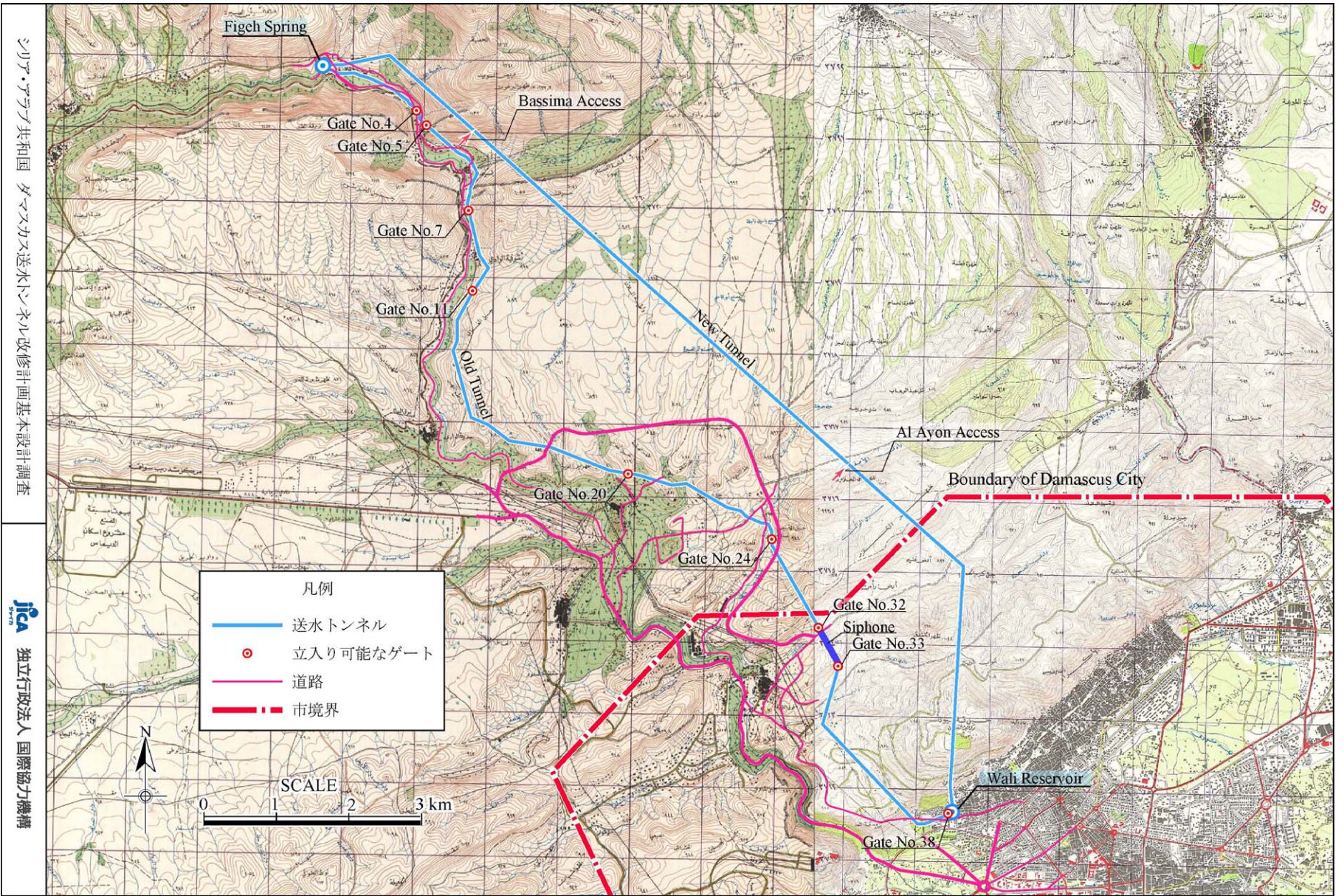
図 2-4 送水トンネル・道路位置図
