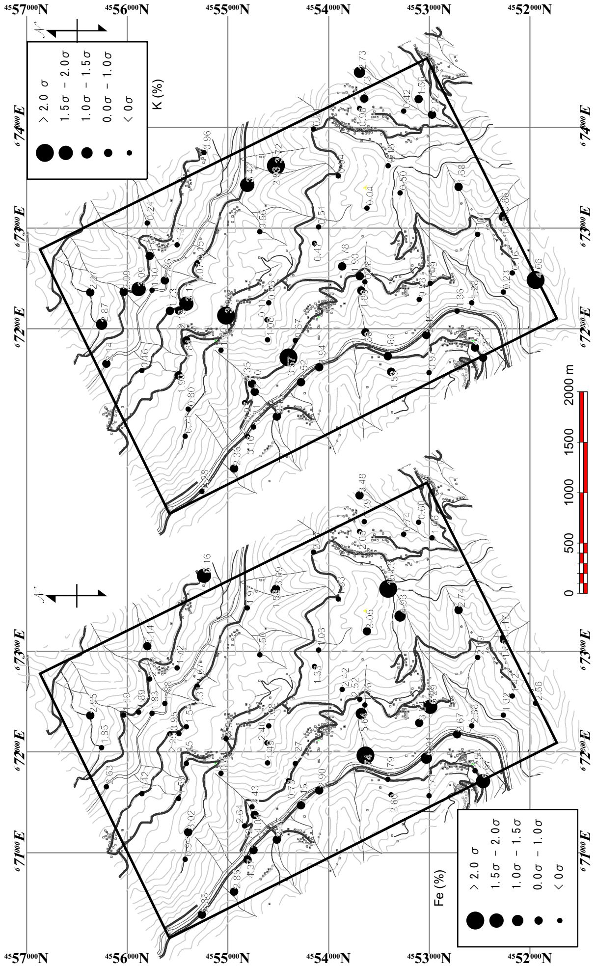
資料6 全岩分析元素別分布図 (Fe,K)
