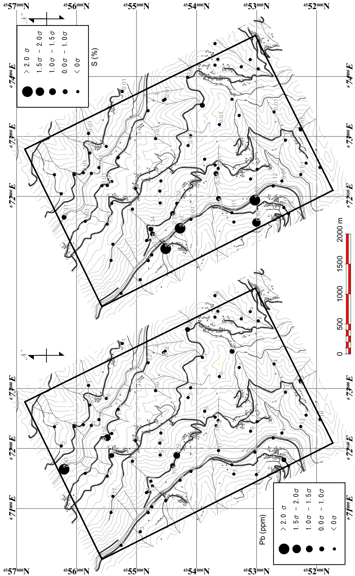
資料6 全岩分析元素別分布図 (Pb,S)
