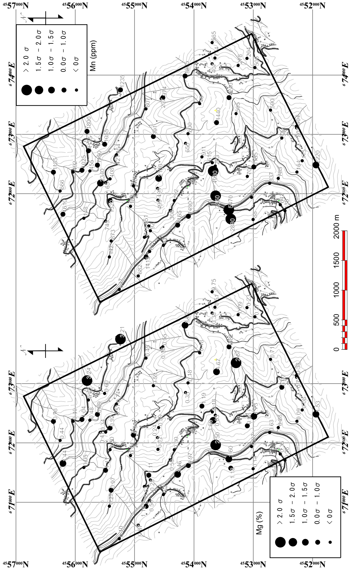
資料6 全岩分析元素別分布図 (Mg,Mn)
