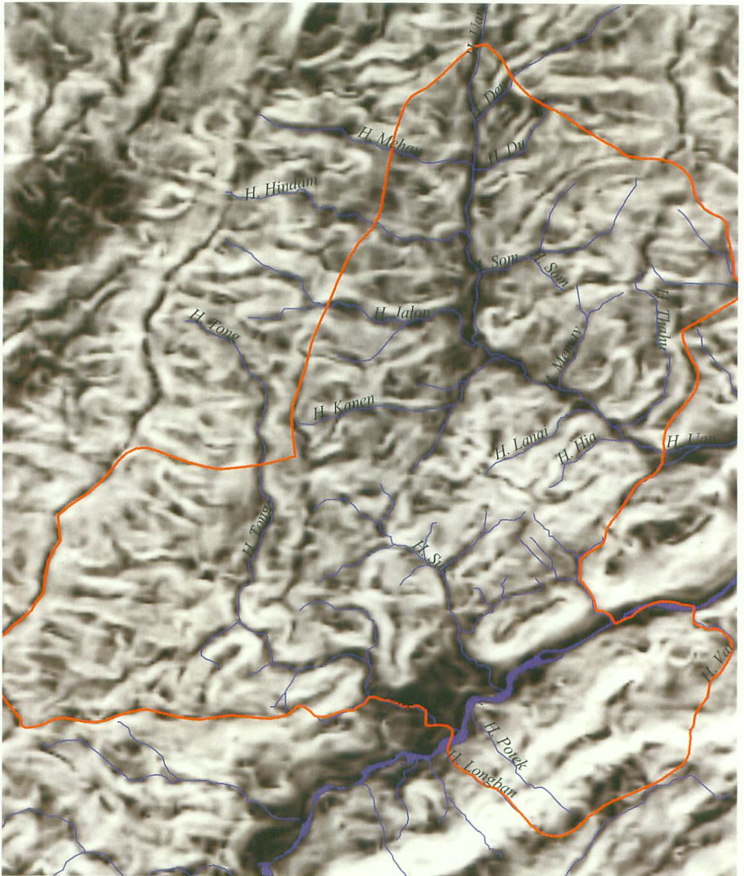
図4 ASTER Slope Image (ハットファイ村)
