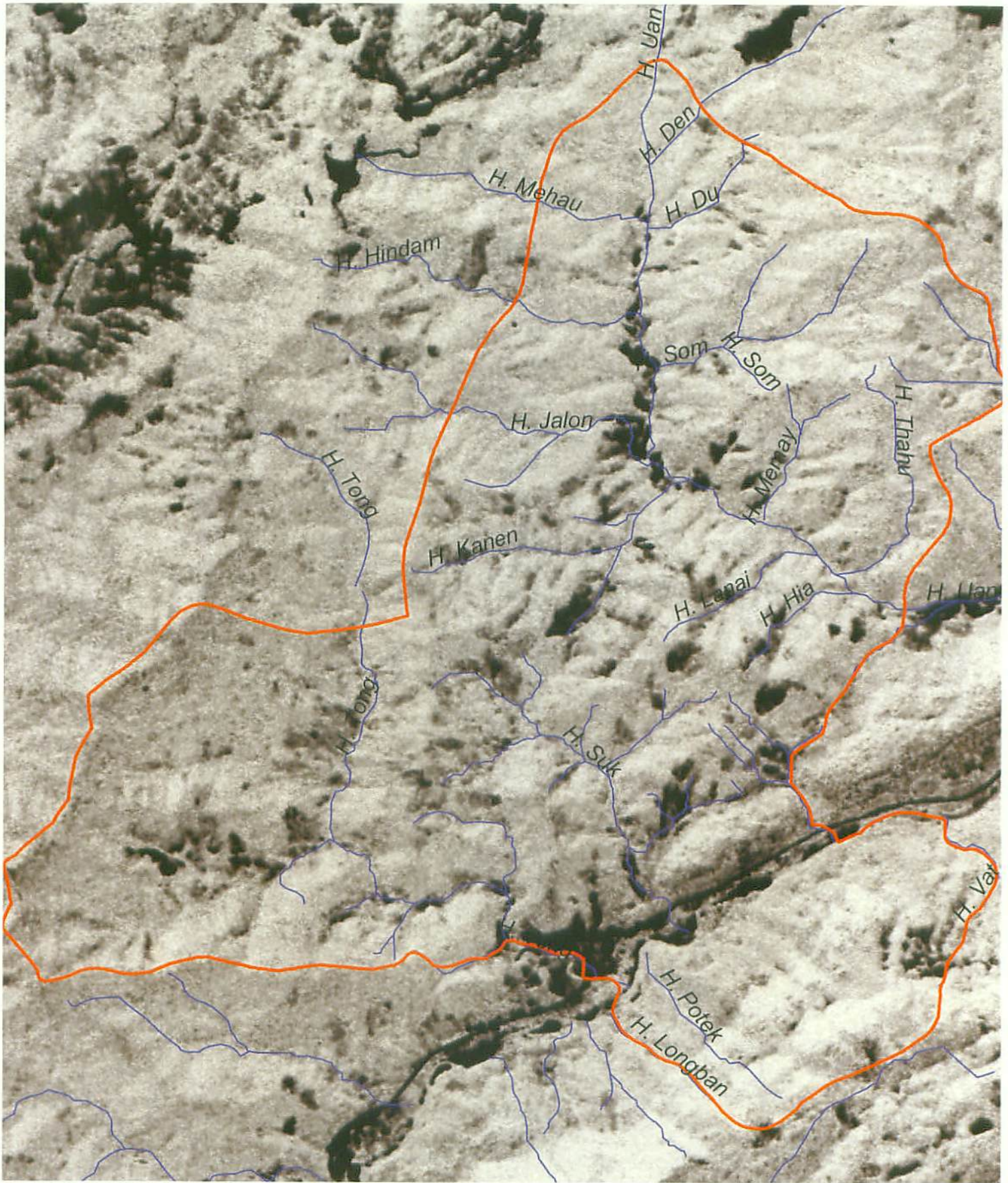
図 3 Normalized Vegetation Index (ハットファイ村)
