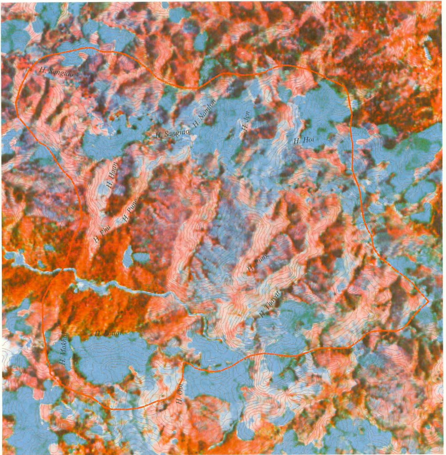
図 10 SPOT False Color Image (サムトン村)
