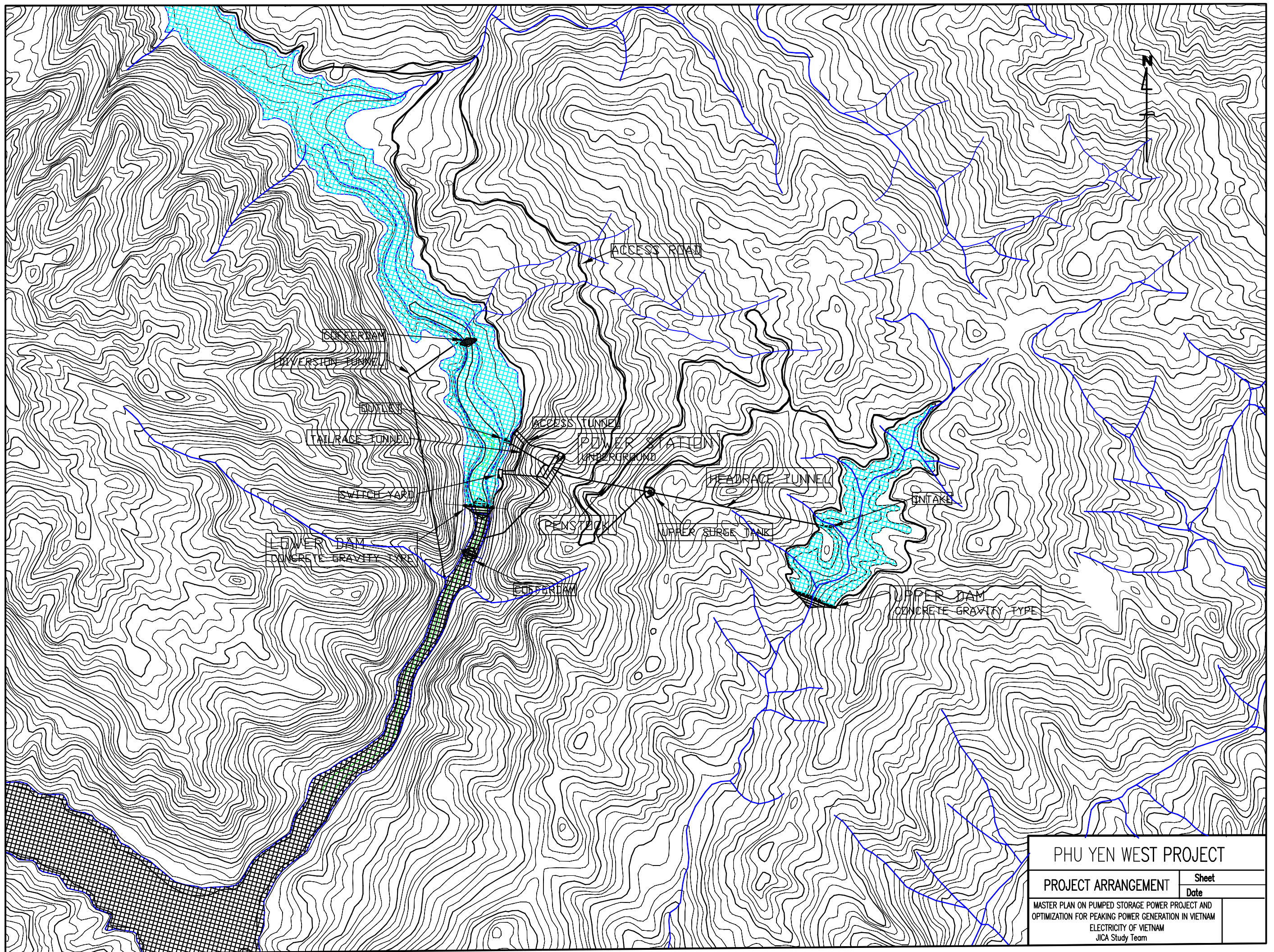
図 4-3-9 Phu Yen West地点の計画平面図
