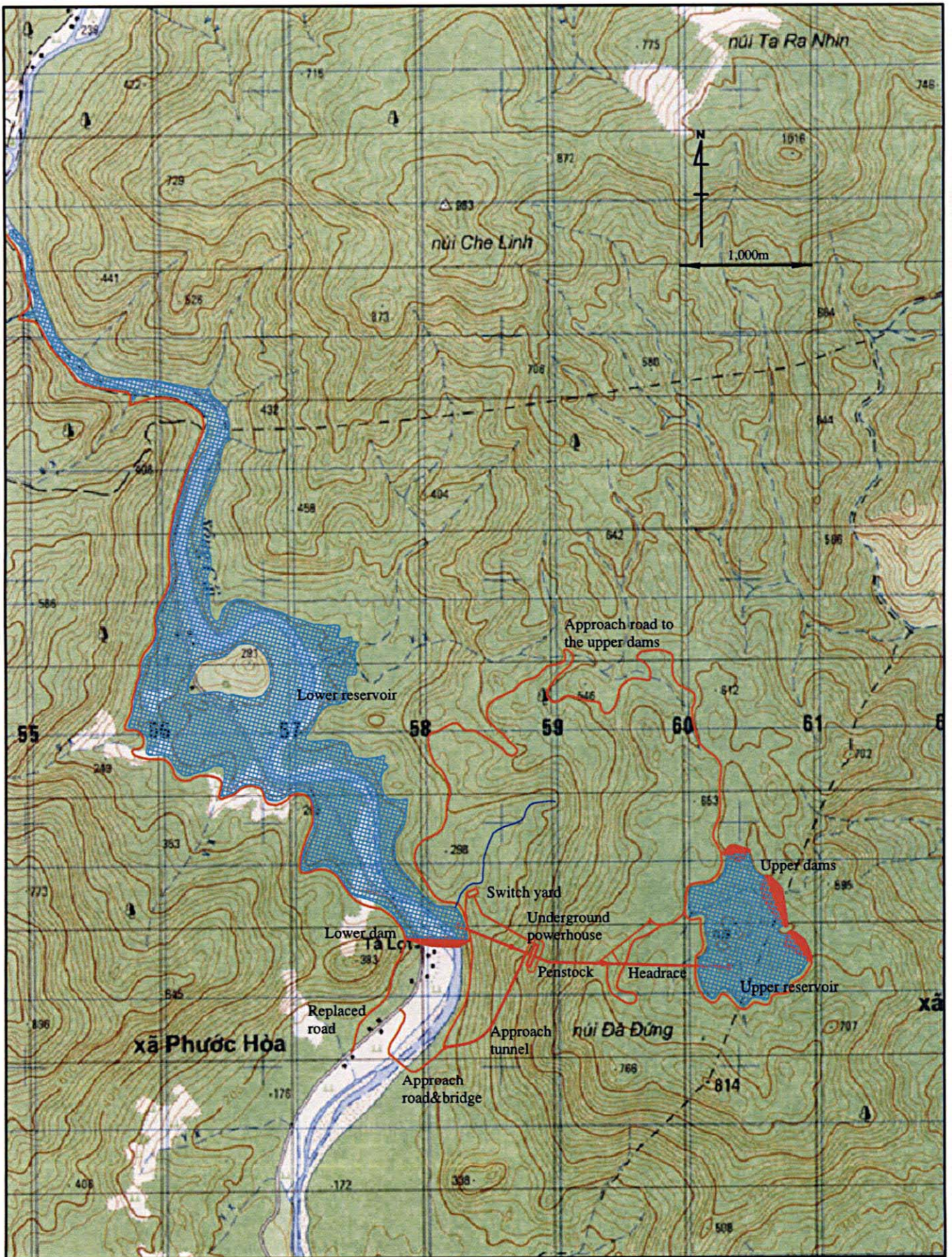
図 4-2-9 Bac Ai (JS6) 地点 概略レイアウト
