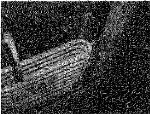
カスンク 県 (Kasungu District) KALULUMA Rural Hospital 冷蔵庫 (ケボンタイプ)
