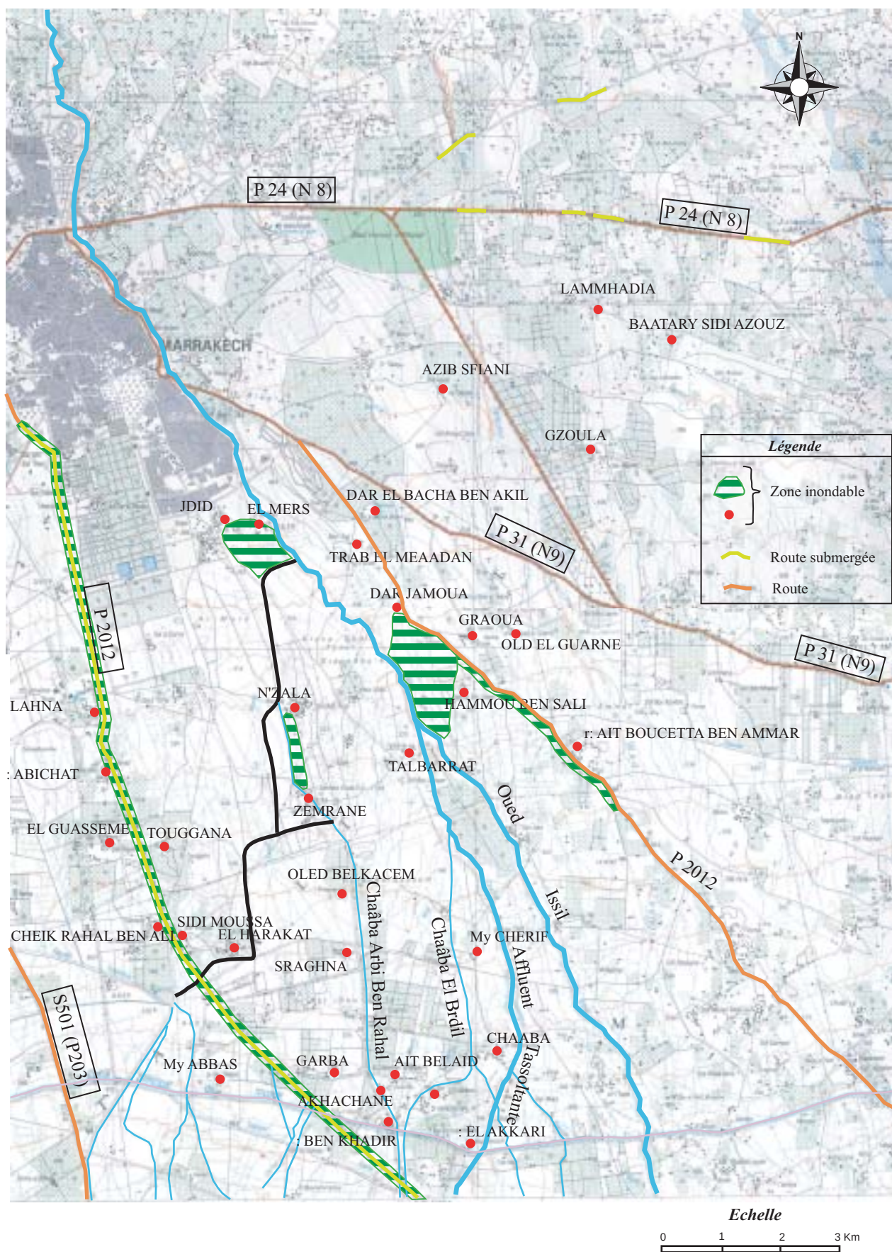
Fig. C.2.1(2/3) CARTE DE CRUE (CRUE DU 27-31/3, 5-8/4/1997)
