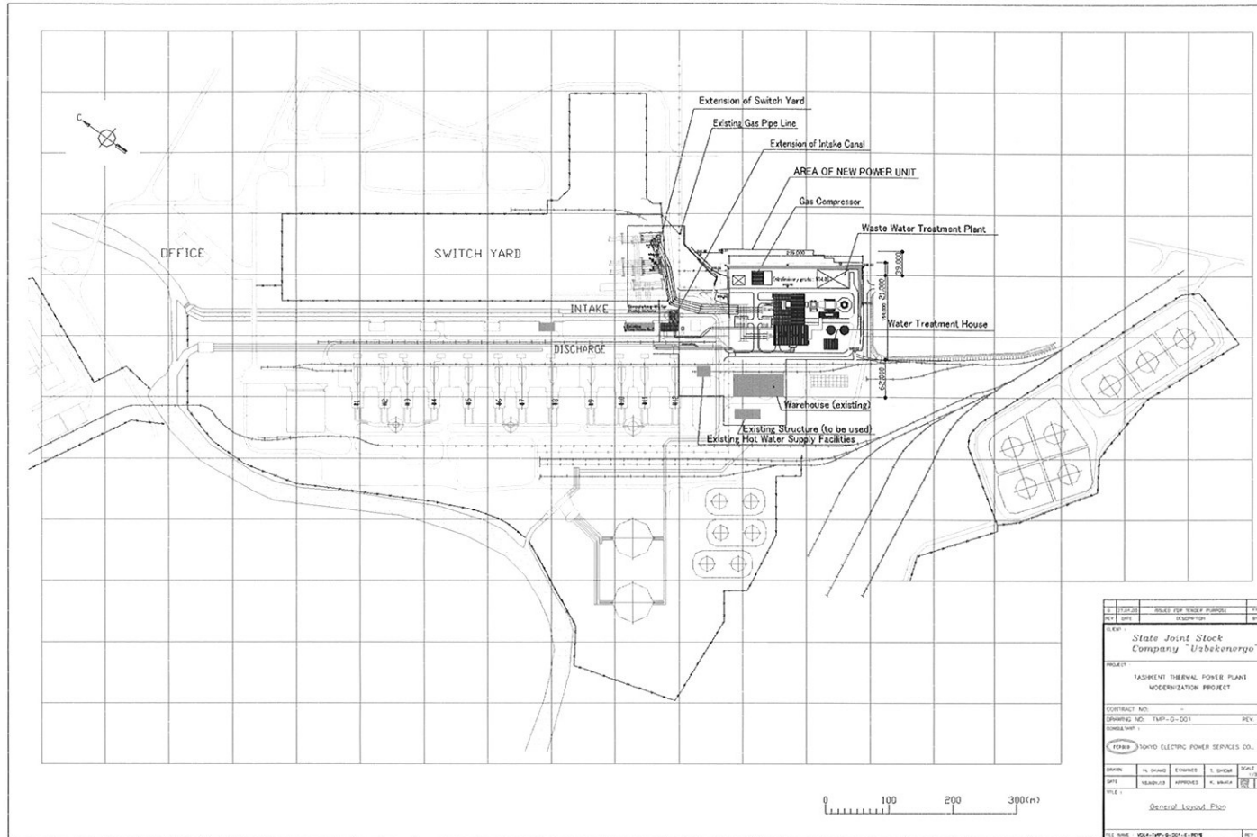
タシケント火力発電所配置図（近代化後）
