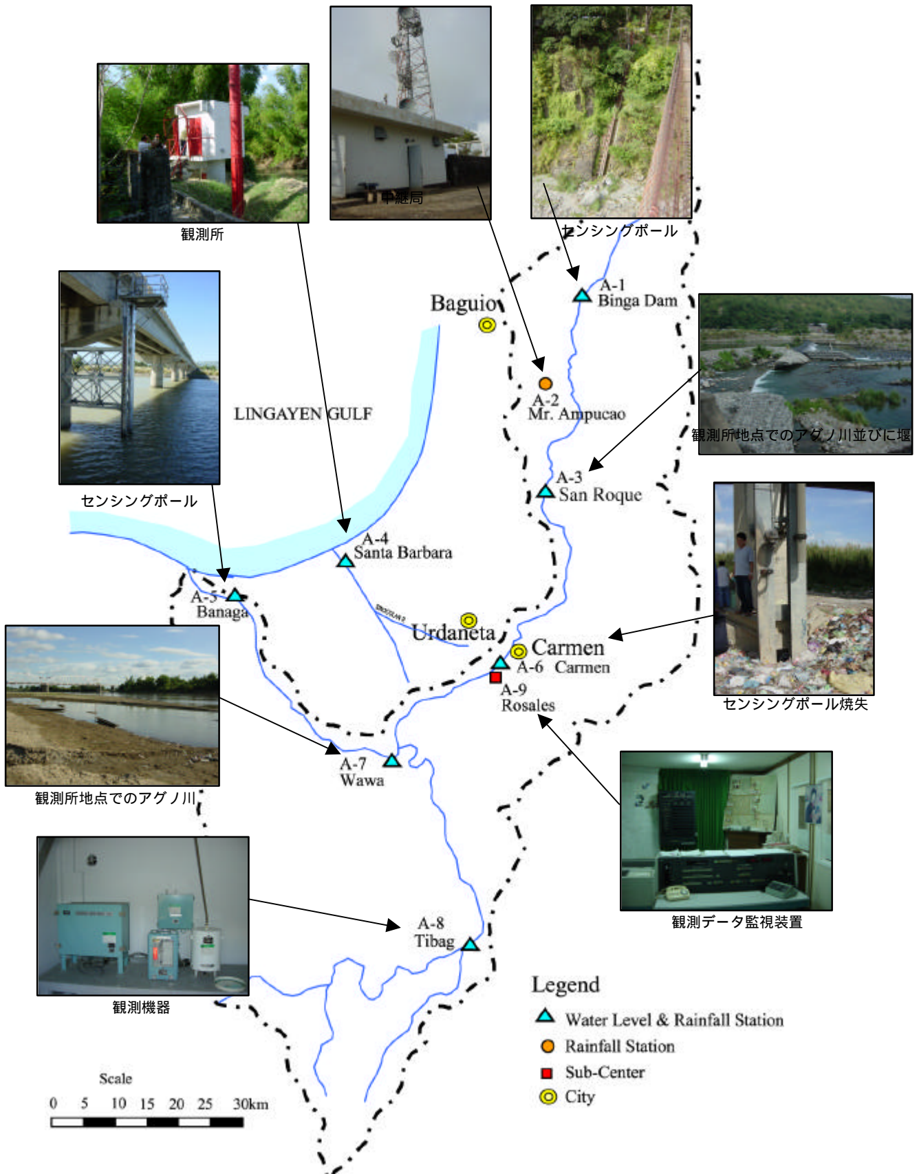
図 - 4 洪水予警報システムの現状 (アグノ河流域)
