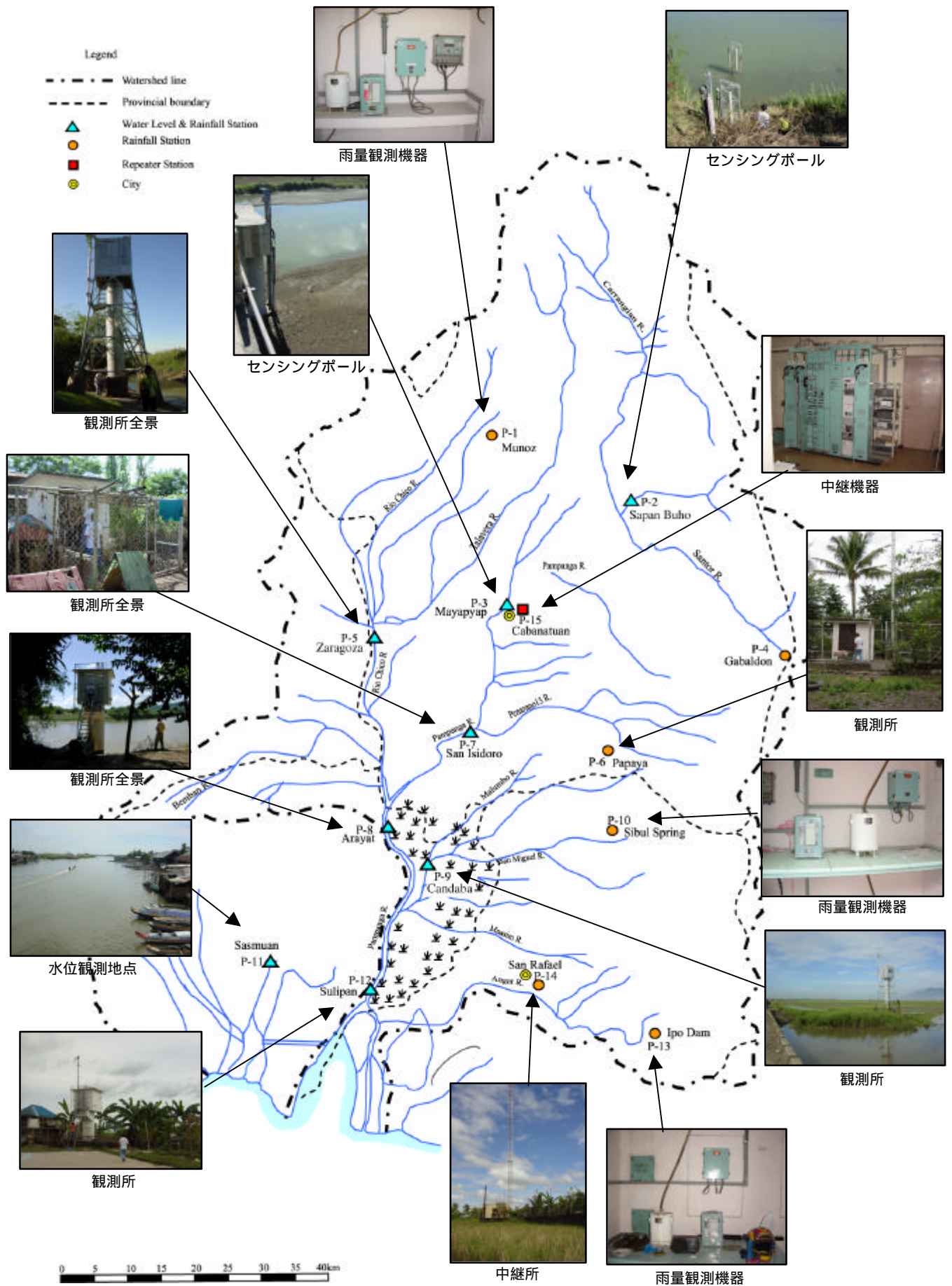
図 - 3 洪水予警報システムの現状 (パンパンガ河流域)
