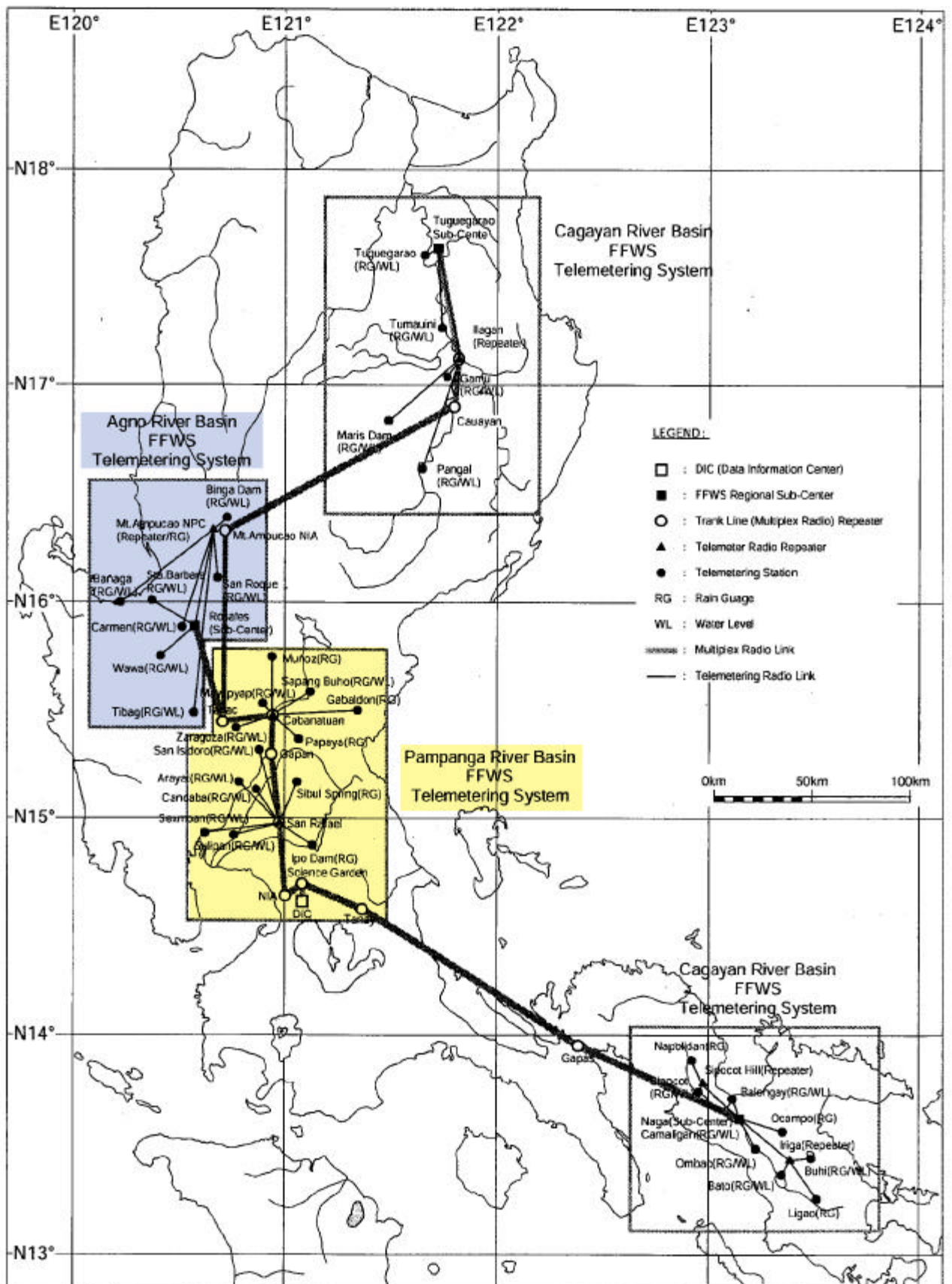
図-2 洪水予警報システム位置図
