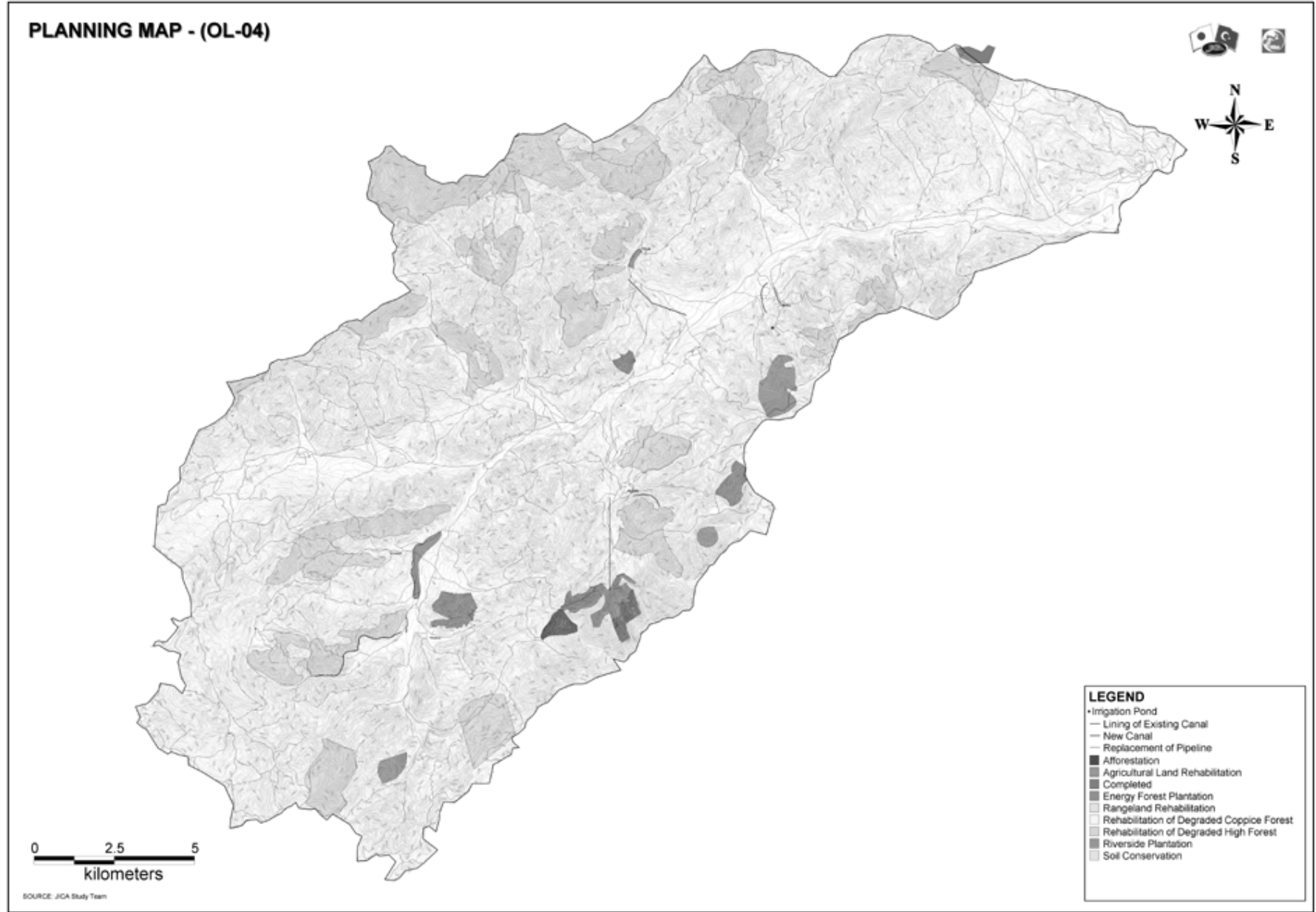
小流域詳細事業計画図(グループ :OL-04)
