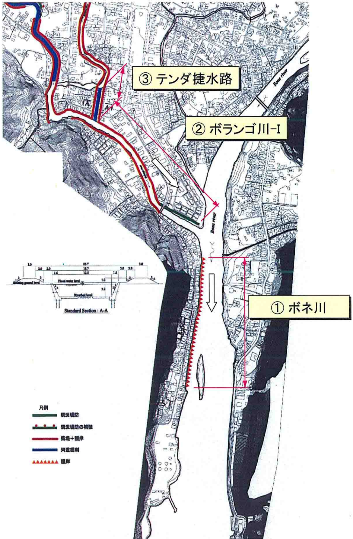
施設計画図 (2)
