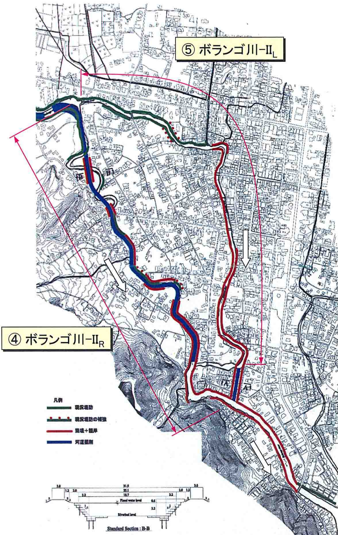
施設計画図 (3)
