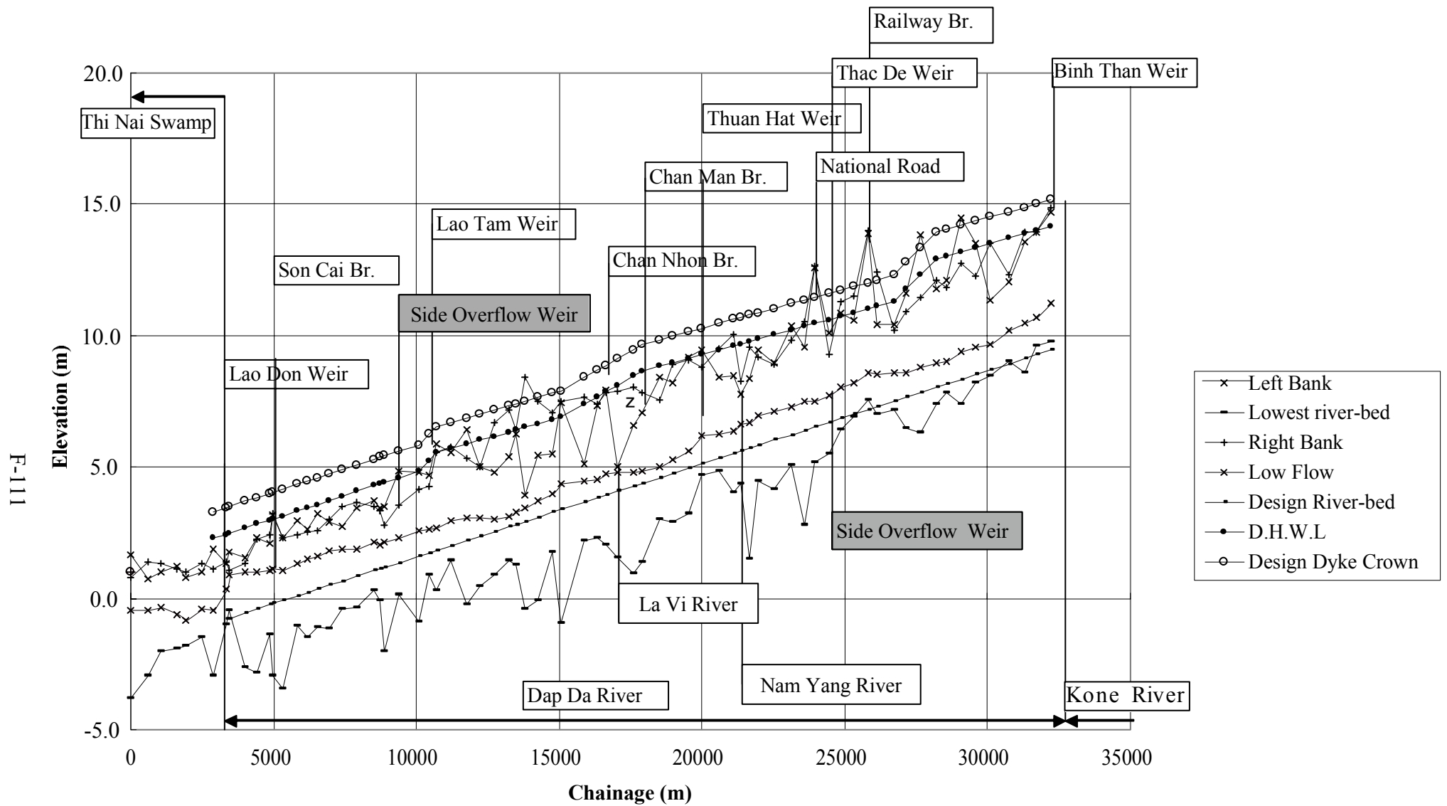
Hình 14.15 Mặt cắt dọc thiết kế của sông Đập Đá với đập tràn bên
