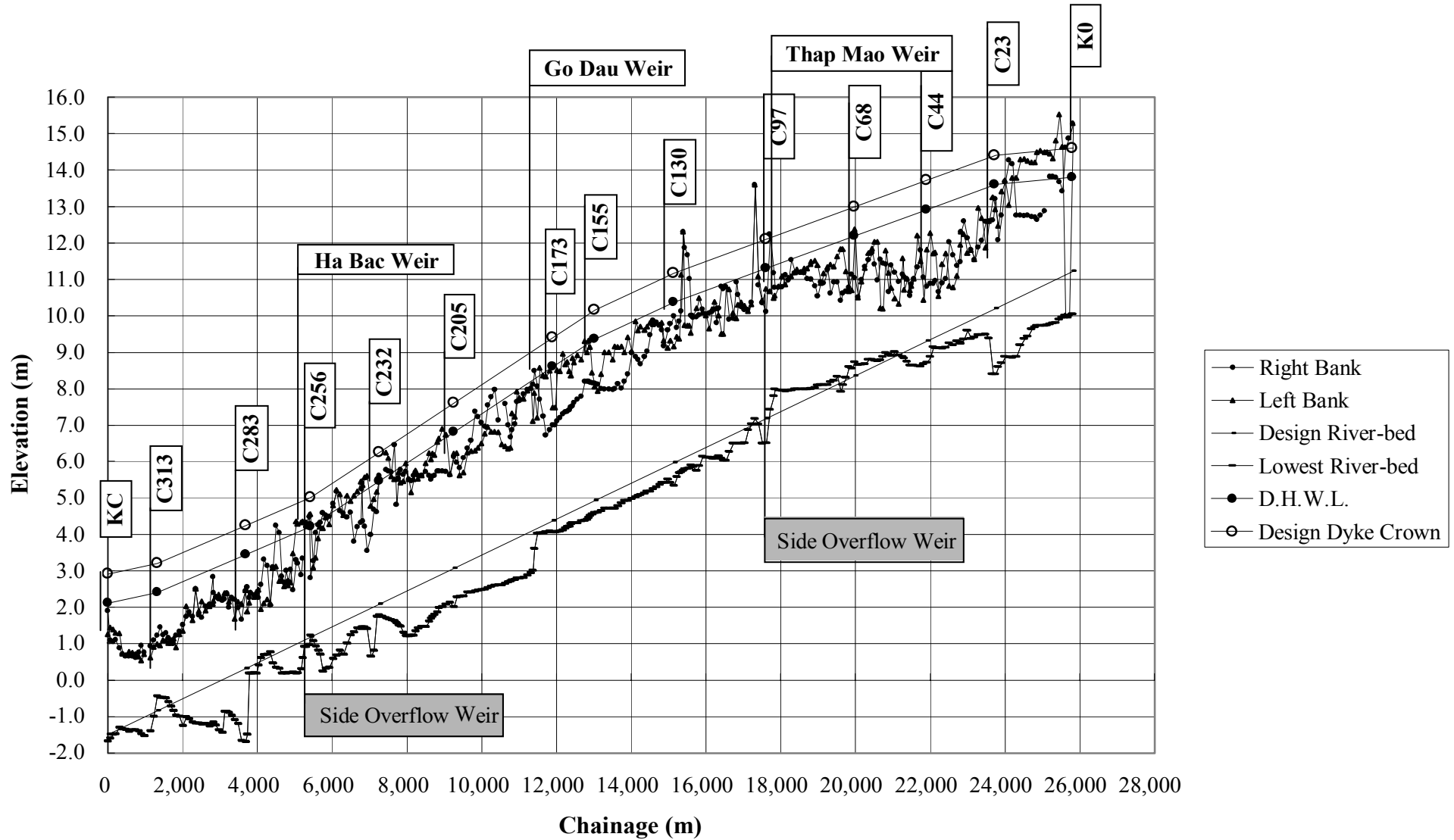
Hình 14.16 Mặt cắt dọc thiết kế của sông Gò Chàm với đập tràn bên
