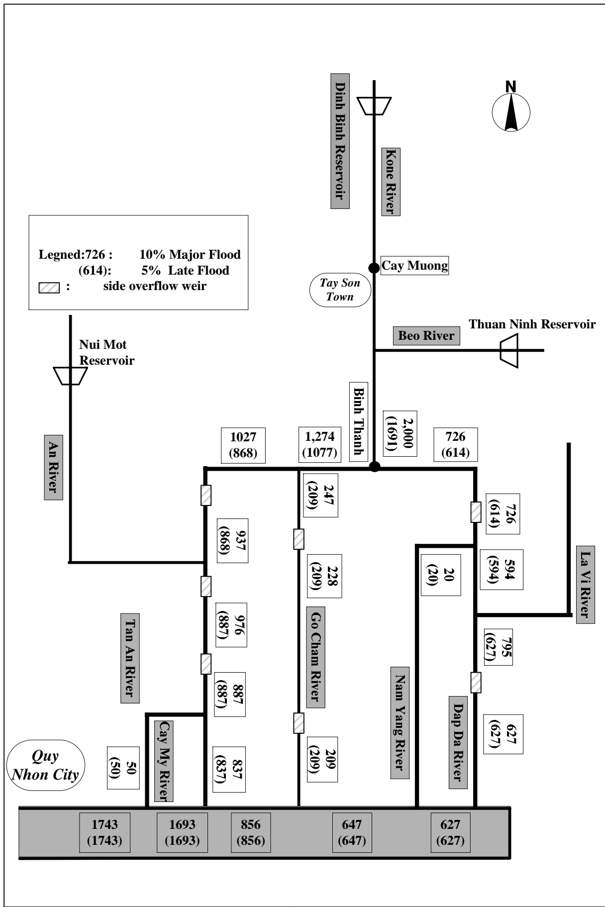
Hình 14.13 Phân bố lưu lượng thiết kế trên lưu vực sông Kone
