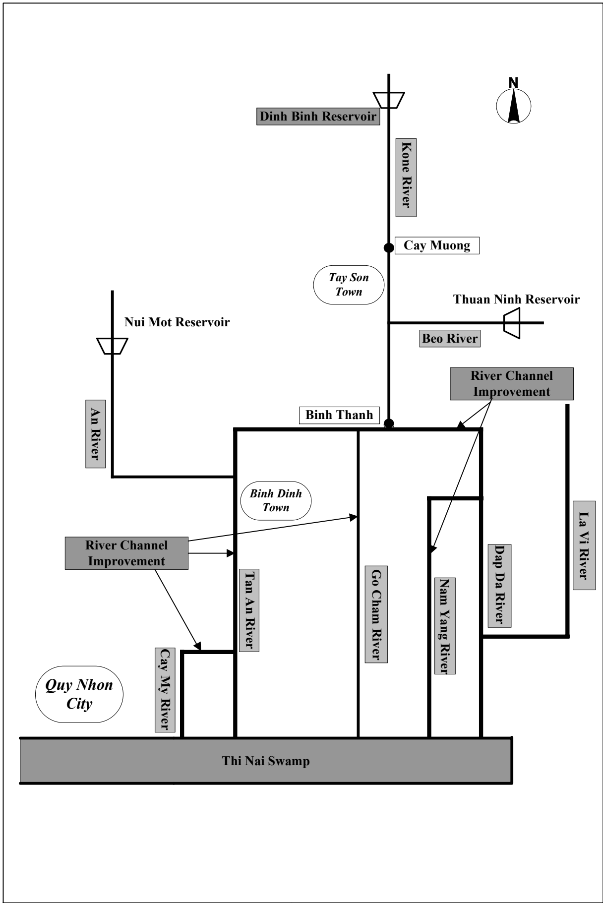
The Study on Nationwide Water Resources Development and Management in the Socialist Republic of Vietnam Hình 7.5 Phân bố các công trình chống lũ của sông Kone JAPAN INTERNATIONAL COOPERATION AGENCY
