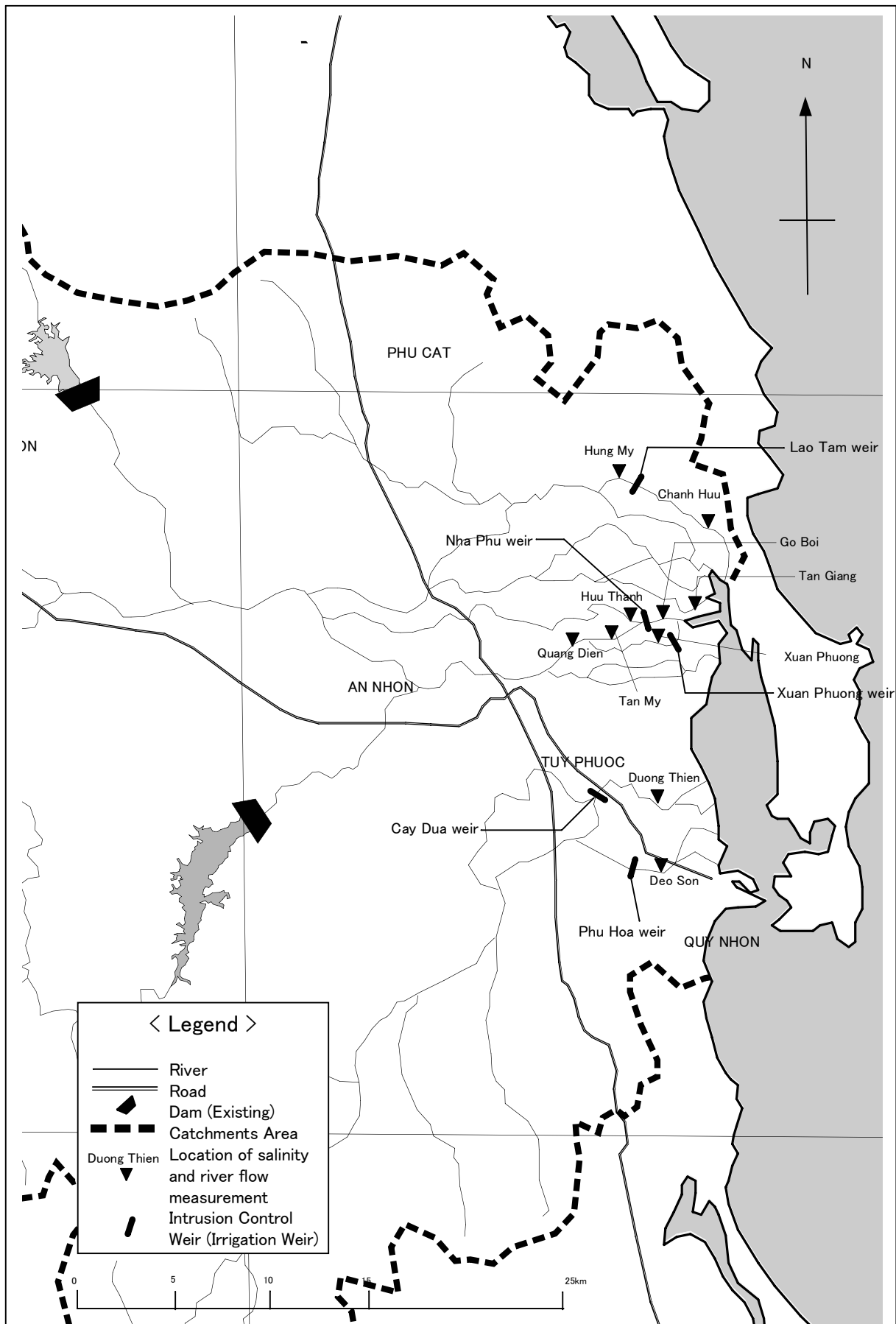
Hình 5.4 Các địa điểm đo lường độ mặn và Đập chống mặn
