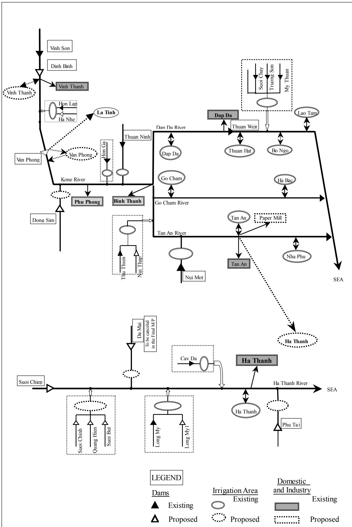
Hình 6.1 Mô hình phân tích cân bằng nước
