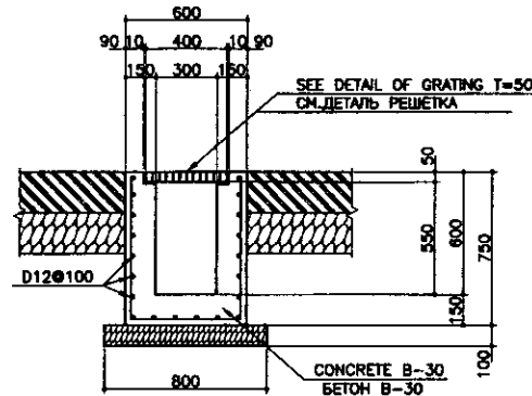
DETAIL (B) / ДЕТАЛЬ (Б)
