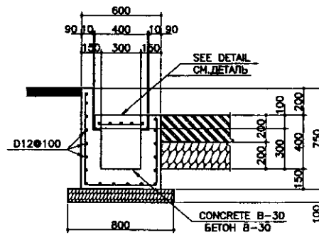
DETAIL (A) / ДЕТАЛЬ (А)
