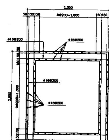
WALL ARRANGEMENT scale 1:30 КОНСТРУКЦИЯ СТЕНЬ
