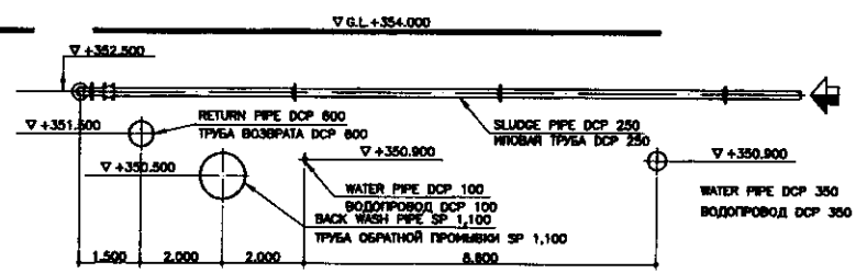
SECTION B-B / ПАЗРЕЗ Б-Б SCALE 1:100
