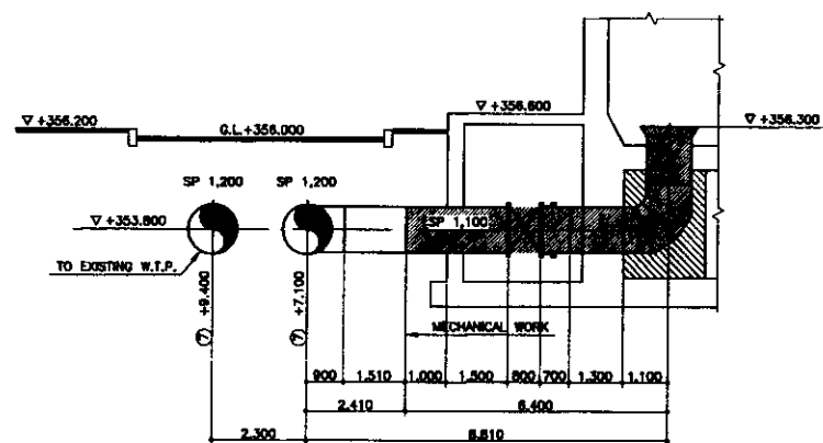
SECTION A-A/РАЗРЕЗ A-A SCALE 1:100
