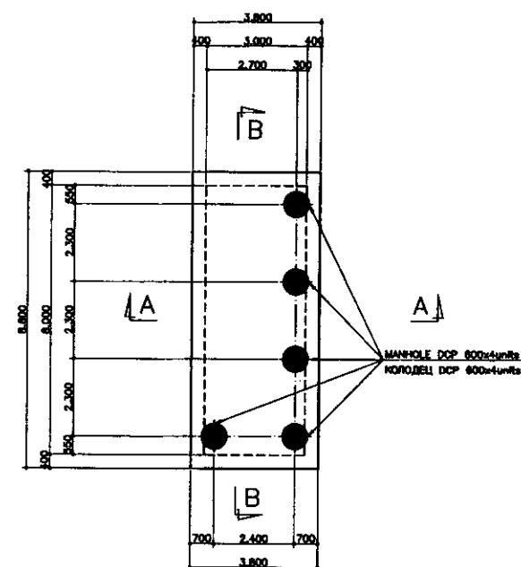
TOP PLAN (Верхний план)
