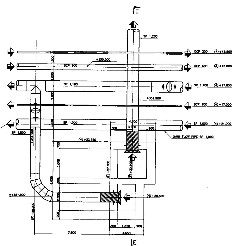
DETAIL G / ДЕТАЛЬ G SCALE 1:100
