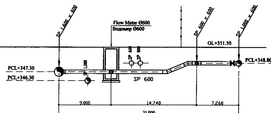
SECTION E-E PA3PE3 E-E
