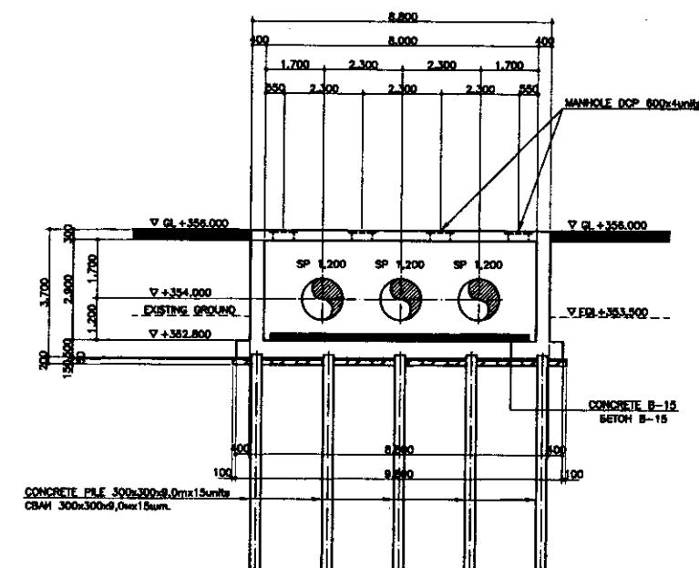
SECTION B-B PA3PE3 B-B
