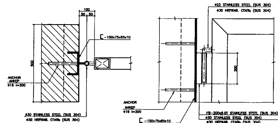
DETAIL B (8 units) ДЕТАЛЬ В (8 ЕДИНИЦ)
