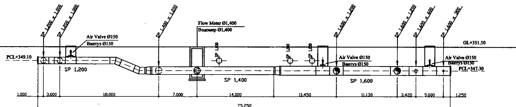
SECTION A-A PA3PE3 A-A
