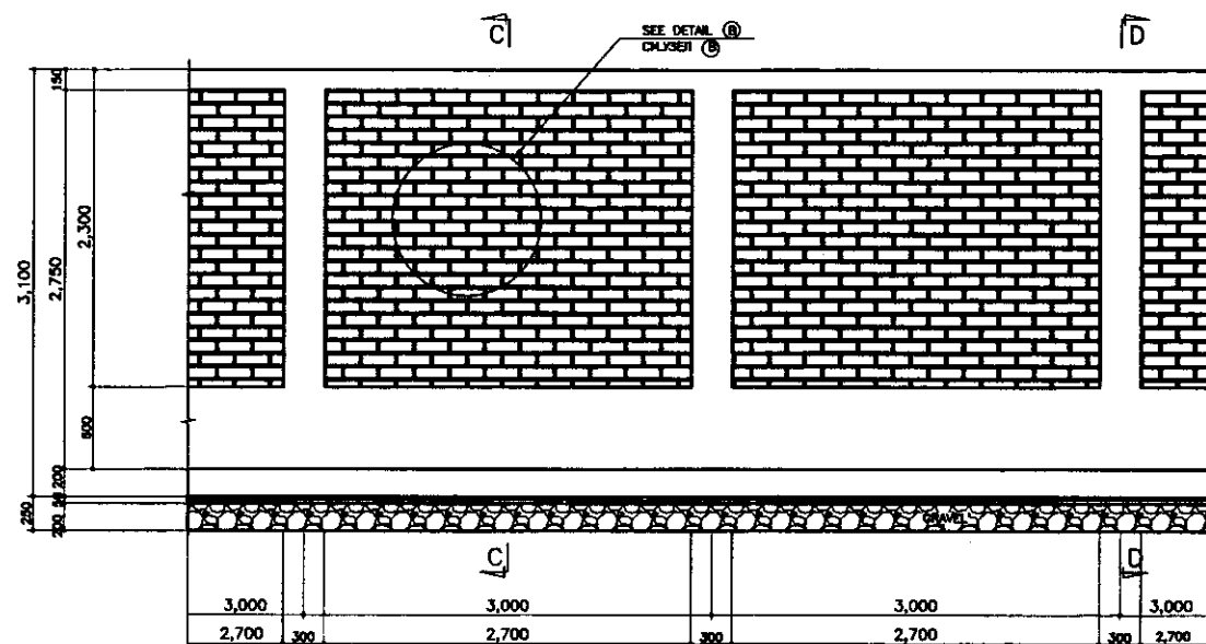
FRONT VIEW ФАСАД SCALE 1:30
