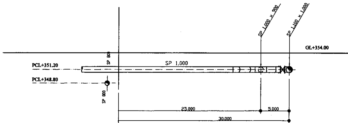
SECTION A-A PA3PE3 A-A
