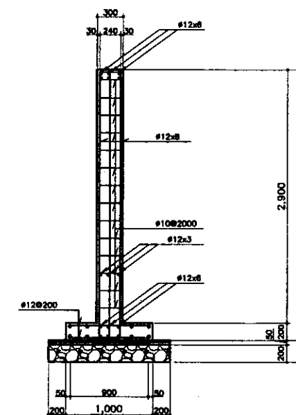
SECTION D-D РАЗРЕЗ D-D SCALE 1:30
