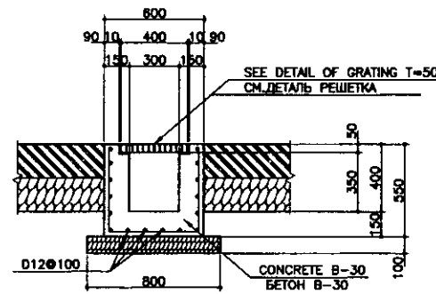
DETAIL (A) / ДЕТАЛЬ (А)
