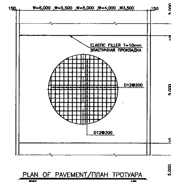
TYPE-2 (W=6,000)/ВИД-2 SCALE 1:50
