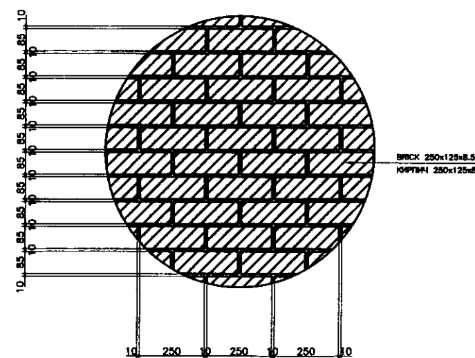
DETAIL B ДЕТАЛЬ B SCALE 1:10
