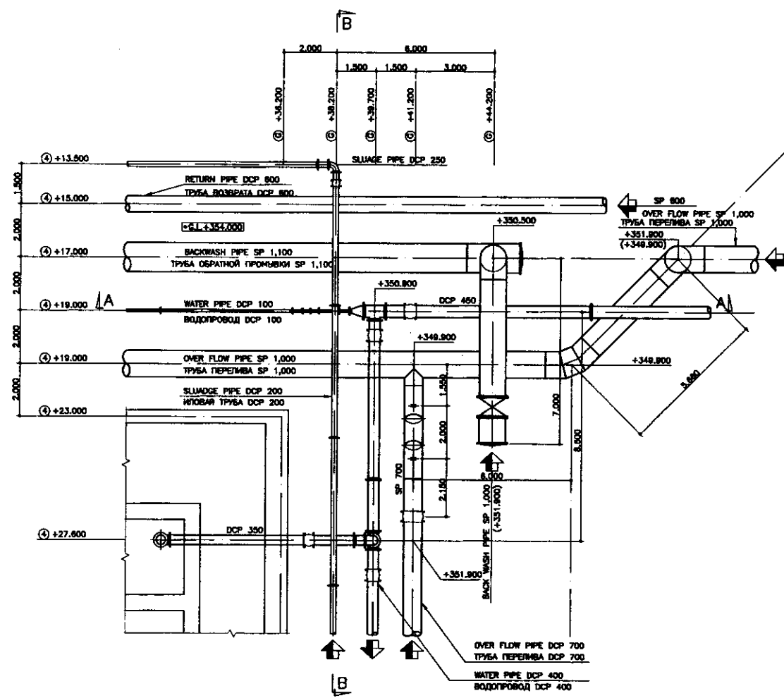
DETAIL (H) / ДЕТАЛЬ (H) SCALE 1:100
