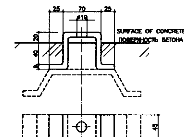
GUIDE RAIL РЕЛЬС-ПРОВОДНИК
