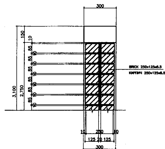
DETAIL A ДЕТАЛЬ A SCALE 1:10
