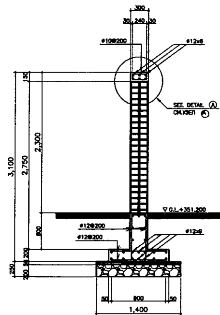
SECTION C-C РАЗРЕЗ C-C SCALE 1:30
