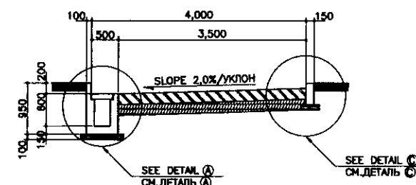
TYPE-6 (W=4,000)/ВИД-6 SCALE 1:50
