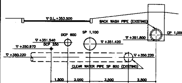
SECTION A-A/PA3PE3 A-A SCALE 1:100
