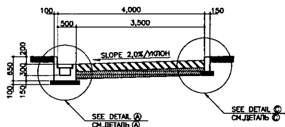
TYPE-4 (W=4,000)/ВИД-4 SCALE 1:50
