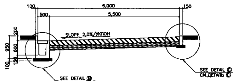
TYPE-3 (W=6,000)/ВИД-3 SCALE 1:50
