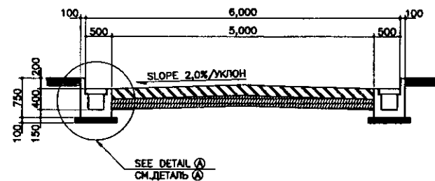
TYPE-1 (W=6,000)/ВИД-1 SCALE 1:50
