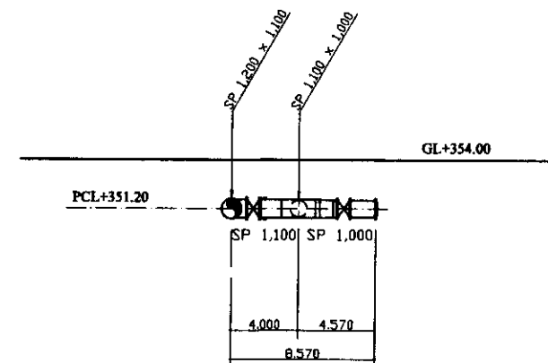
SECTION C-C PA3PE3 C-C
