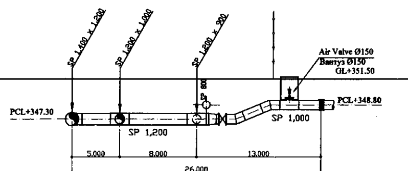
SECTION C-C PA3PE3 C-C
