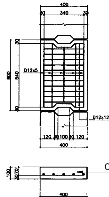
CONCRETE COVER / ЗАЩИТНЫЙ СЛОЙ БЕТОНА
