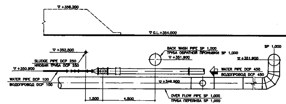
SECTION A-A / ПАЗРЕЗ А-А SCALE 1:100
