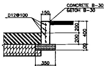
CURB DETAIL (C) / ДЕТАЛЬ БАРДЮРА (С)
