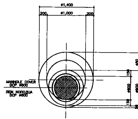
TOP PLAN ВЕРХНИЙ ПЛАН SCALE 1:30
