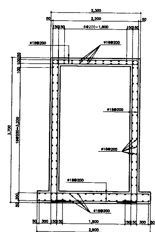
BAR ARRANGEMENT A-A scale 1:30 КОНСТРУКЦИЯ АРМАТУРЫ А-А
