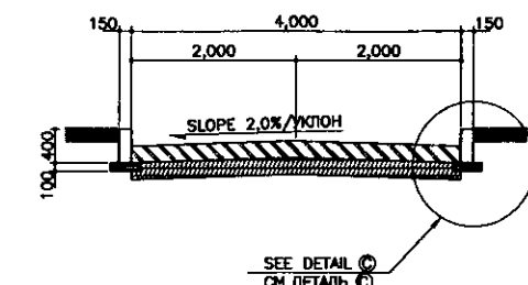
TYPE-5 (W=4,000)/ВИД-5 SCALE 1:50
