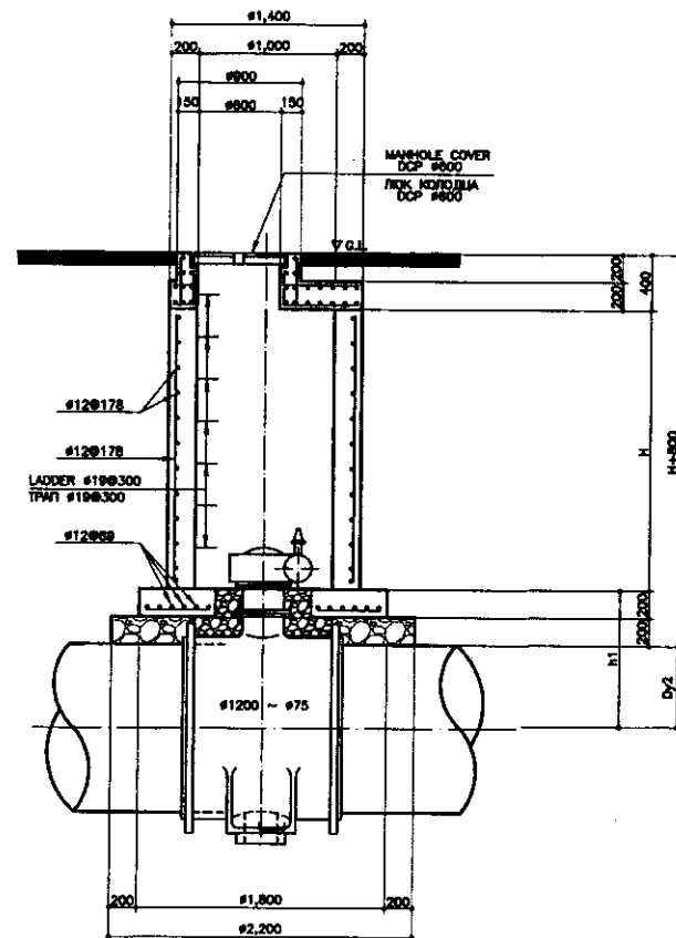
SECTION C-C РАЗРЕЗ С-С SCALE 1:30
