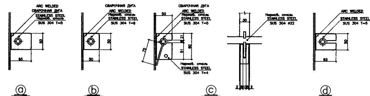
DETAIL A (1 units) ДЕТАЛЬ А (1 единица)
