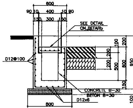
DETAIL (B) / ДЕТАЛЬ (Б)
