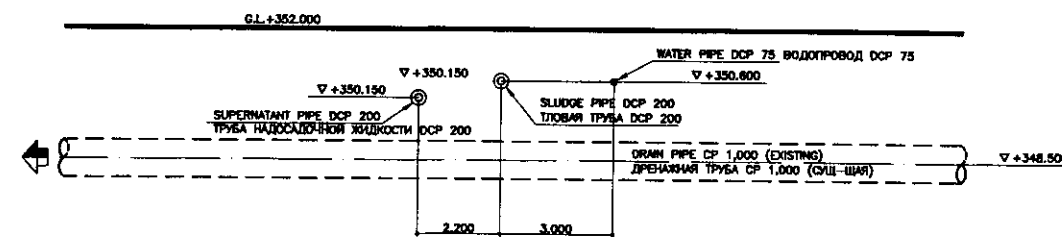
SECTION B-B / РАЗРЕЗ B-B SCALE 1:100
