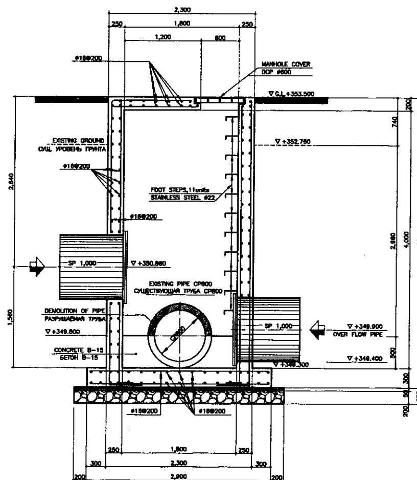
SECTION A-A SCALE 1:30
