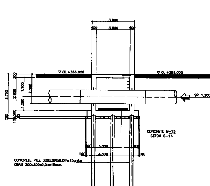
SECTION A-A PA3PE3 A-A
