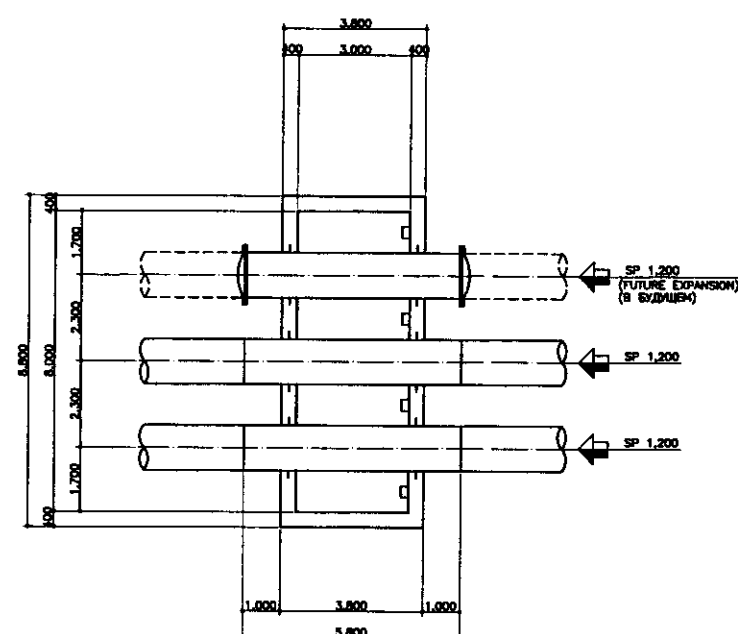
MIDDLE PLAN (средний план)
