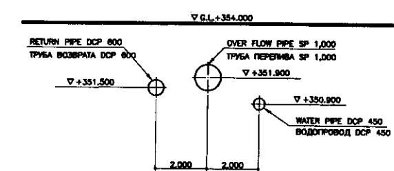
SECTION C-C / ПАЗРЕЗ С-С SCALE 1:100
