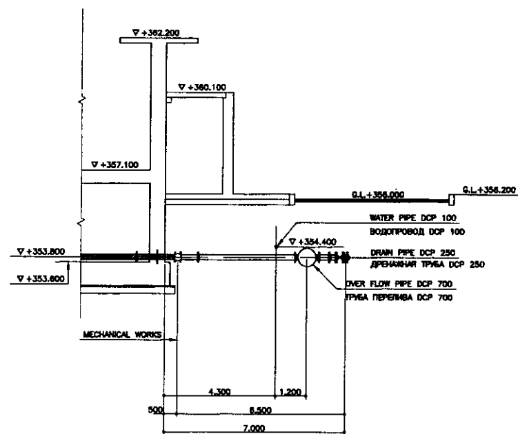
SECTION A-A / РАЗРЕЗ A-A SCALE 1:100
