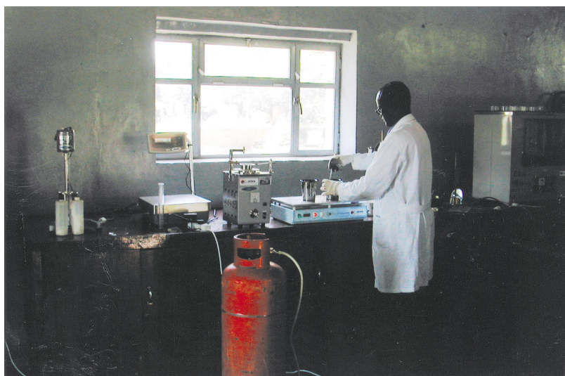
道路保守関連試験機器を用いて試験中のC/P
