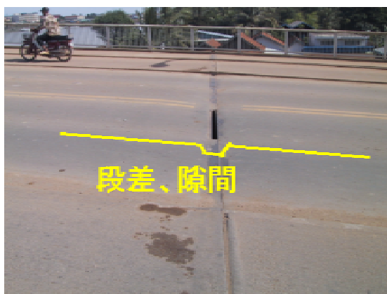
PC 橋梁部伸縮装置・舗装状況
