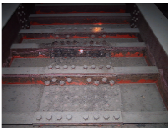
2 径間鋼橋継ぎ手部の錆の発生
