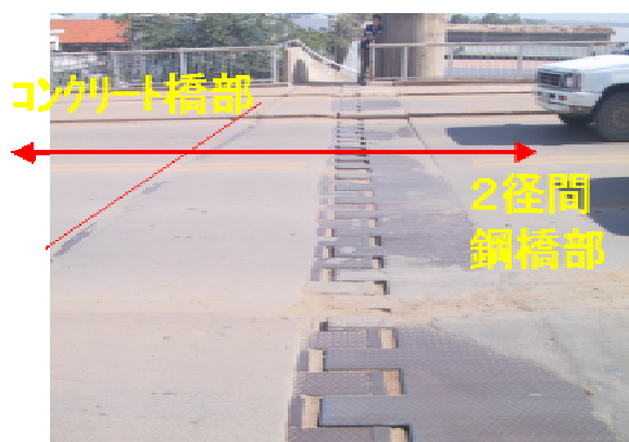
2 径間鋼橋部伸縮装置
