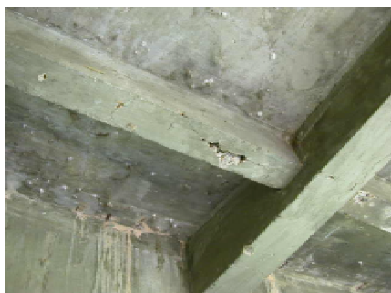
床版横梁のひびわれ
