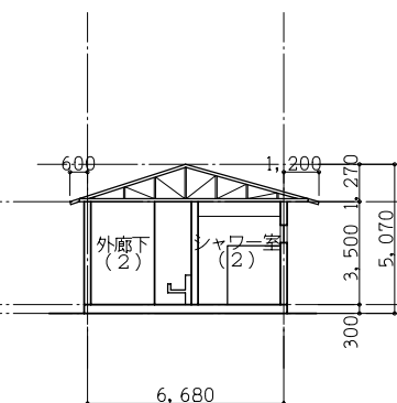
断面図2
