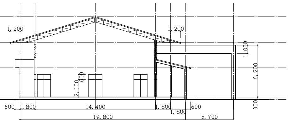
断面図
