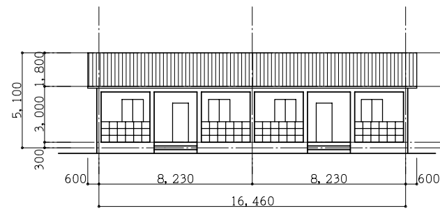
東立面図
