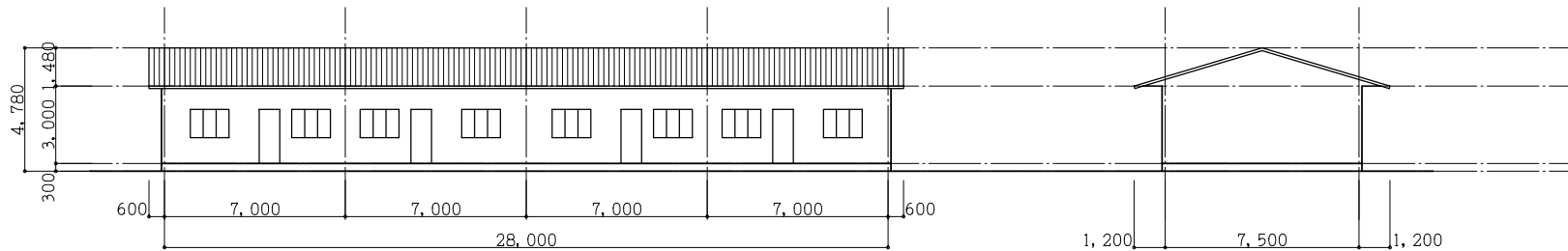
東立面図
