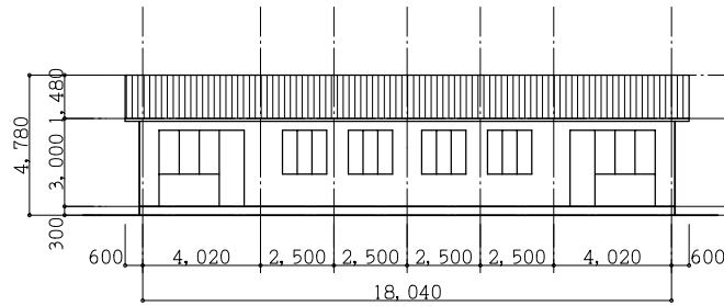
東立面図
