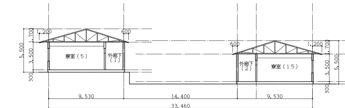
断面図1
