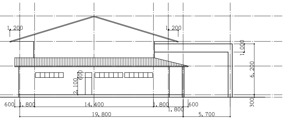
南立面図
