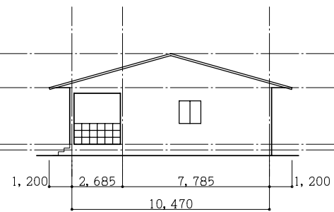
北立面図
