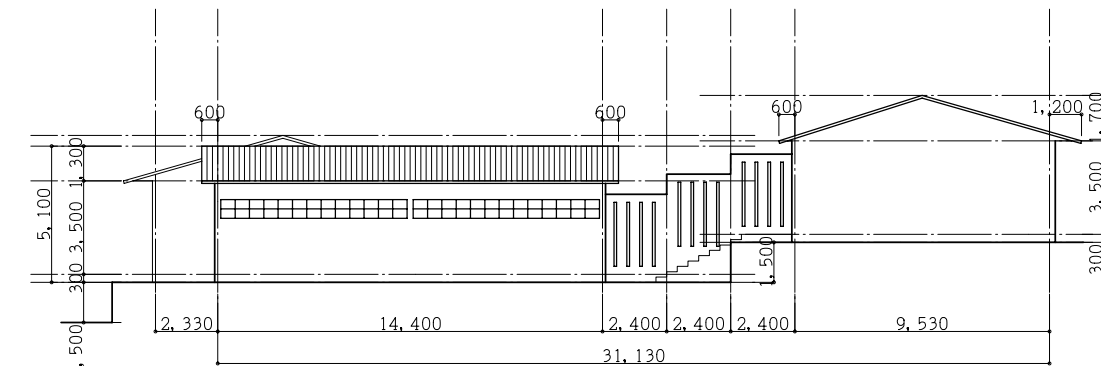
南立面図
