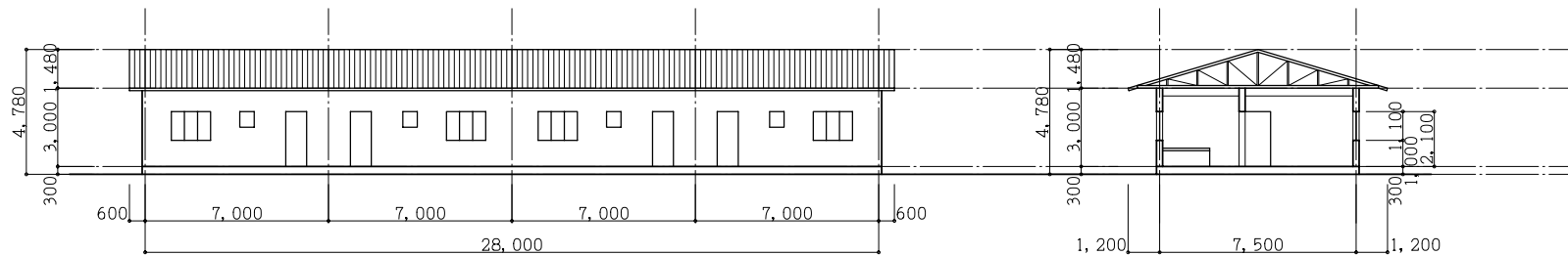
西立面図
