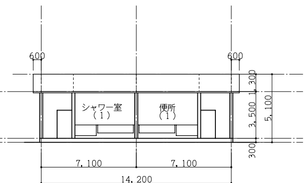
断面図3
