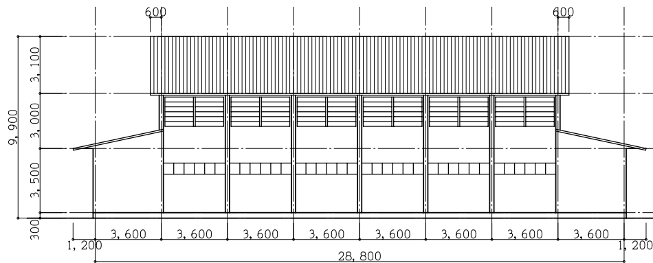
西立面図
