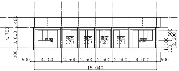
断面図
