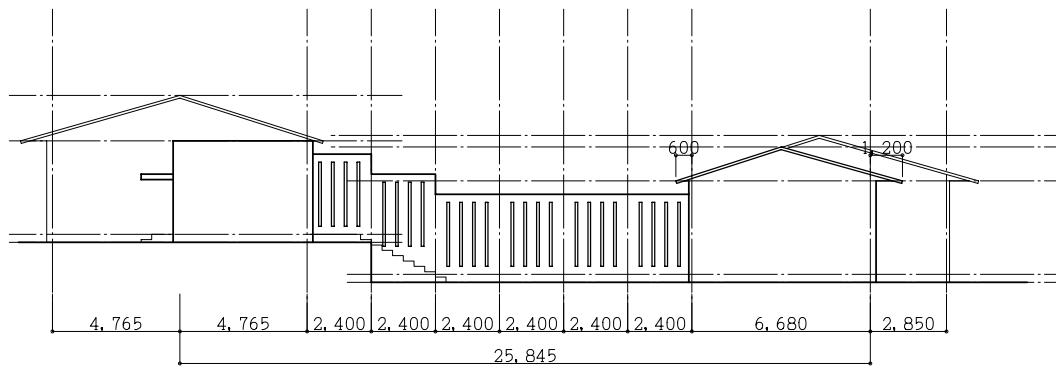
北立面図
