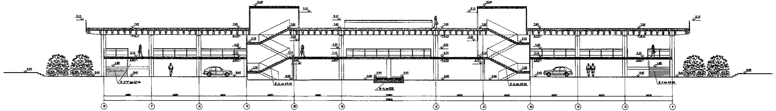
Павильон - 1, разрез 4-4
