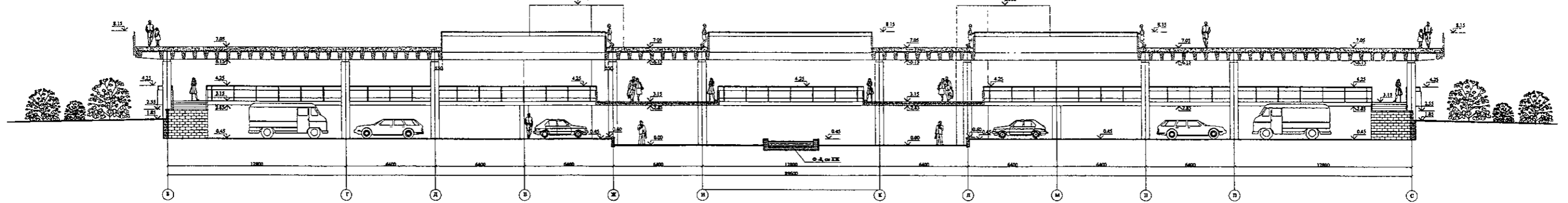
Павильон - 2, разрез 2-2
