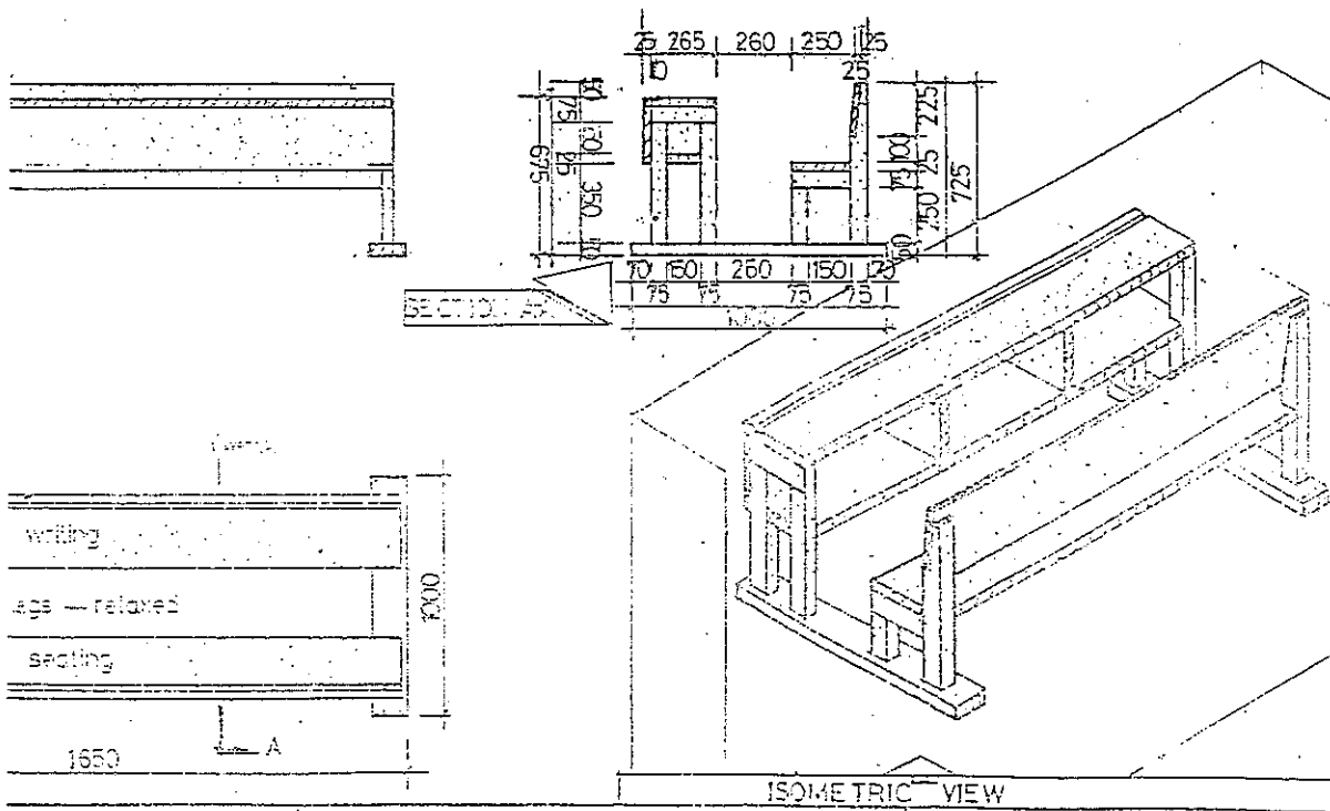
生徒用机・椅子 (3人掛け、木製) 資料: SPEB, カドゥナ州)
