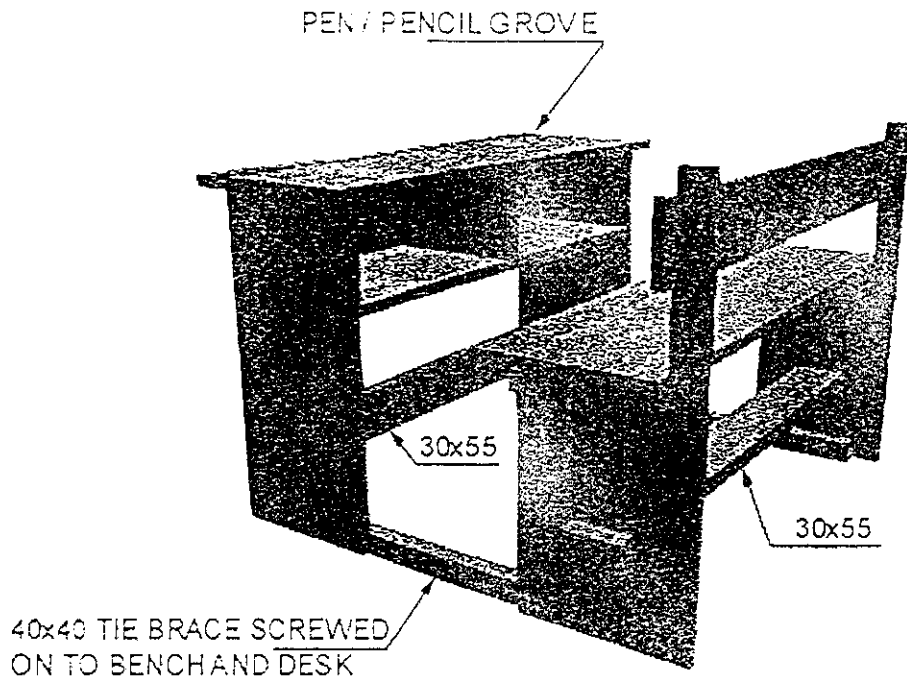
生徒用机・椅子 (2人掛け、木製) 資料: SPEB, ナイジャー州)
