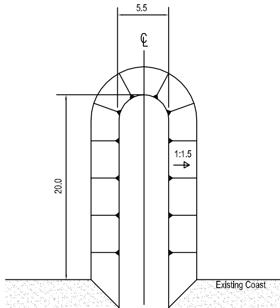
Jetty - Plan
