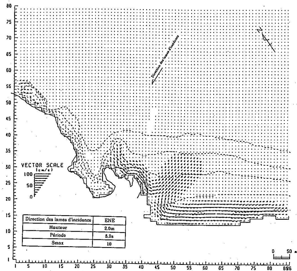
Figure 2.2-4(1) Résultat du calcul du courant littoral (Topographie actuelle, direction du vent : ENE)
