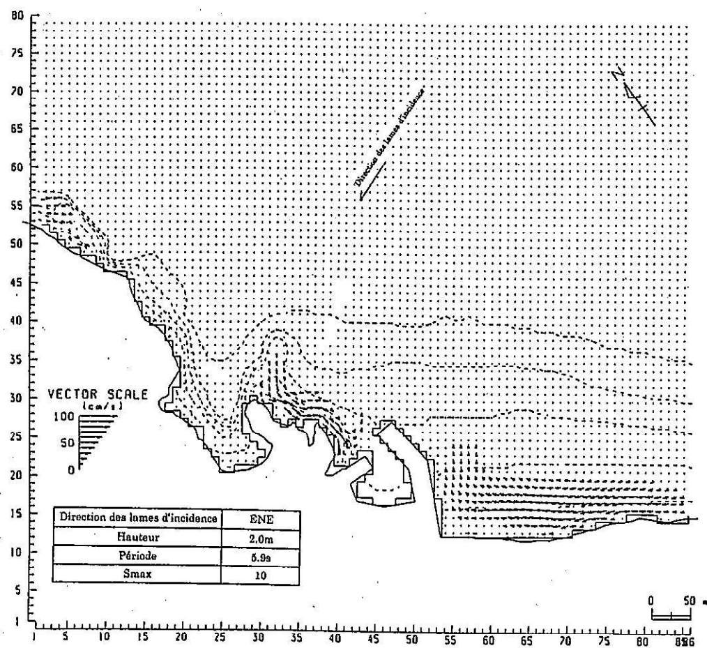
Figure 2.2-5(1) Résultat du calcul du courant littoral (Après la réalisation du port de pêche, direction du vent : ENE)
