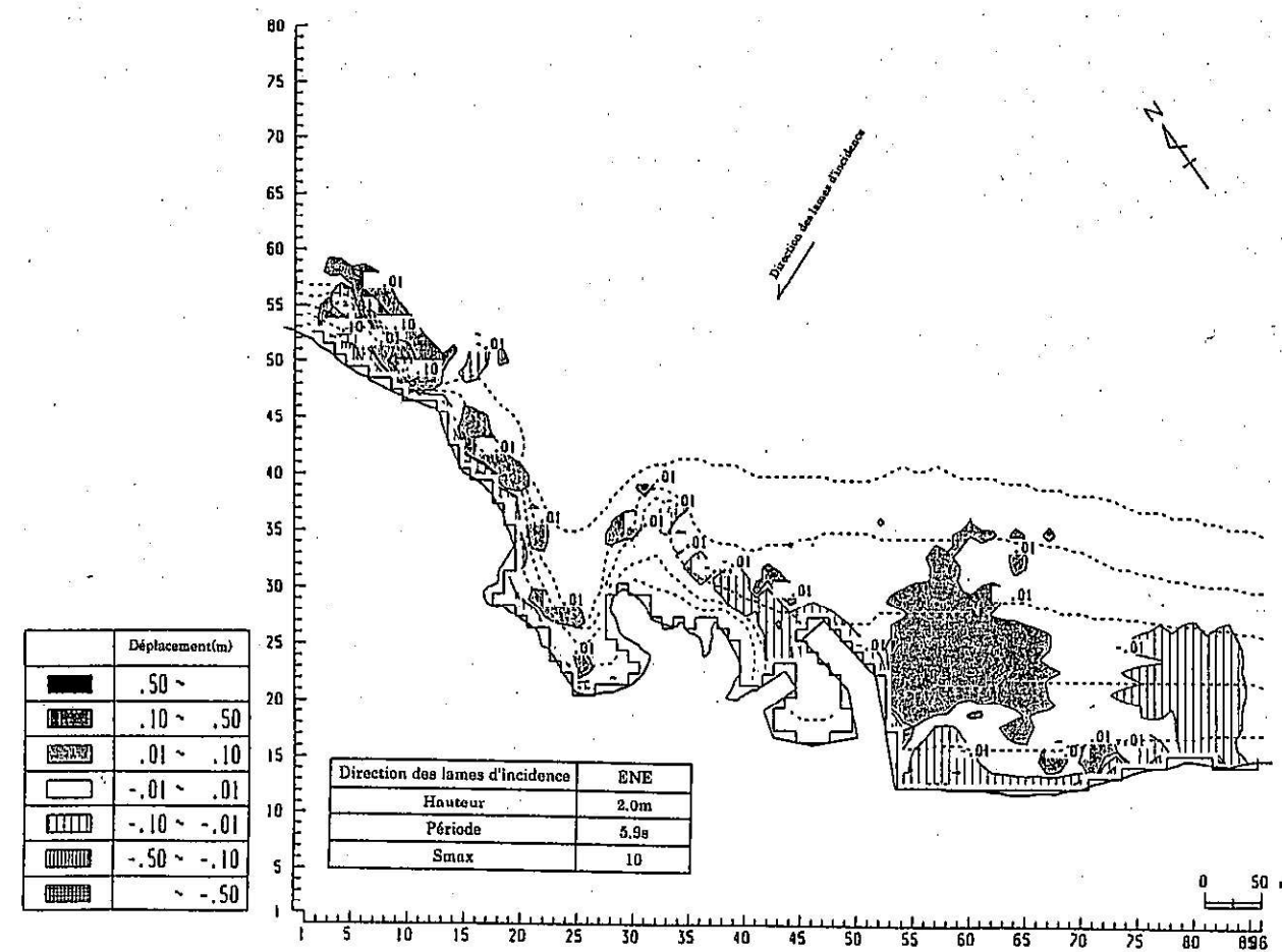
Figure 2.2-5(2) Résultat de la prédiction du changement topographique (Après la réalisation du port de pêche, direction du vent : ENE)
