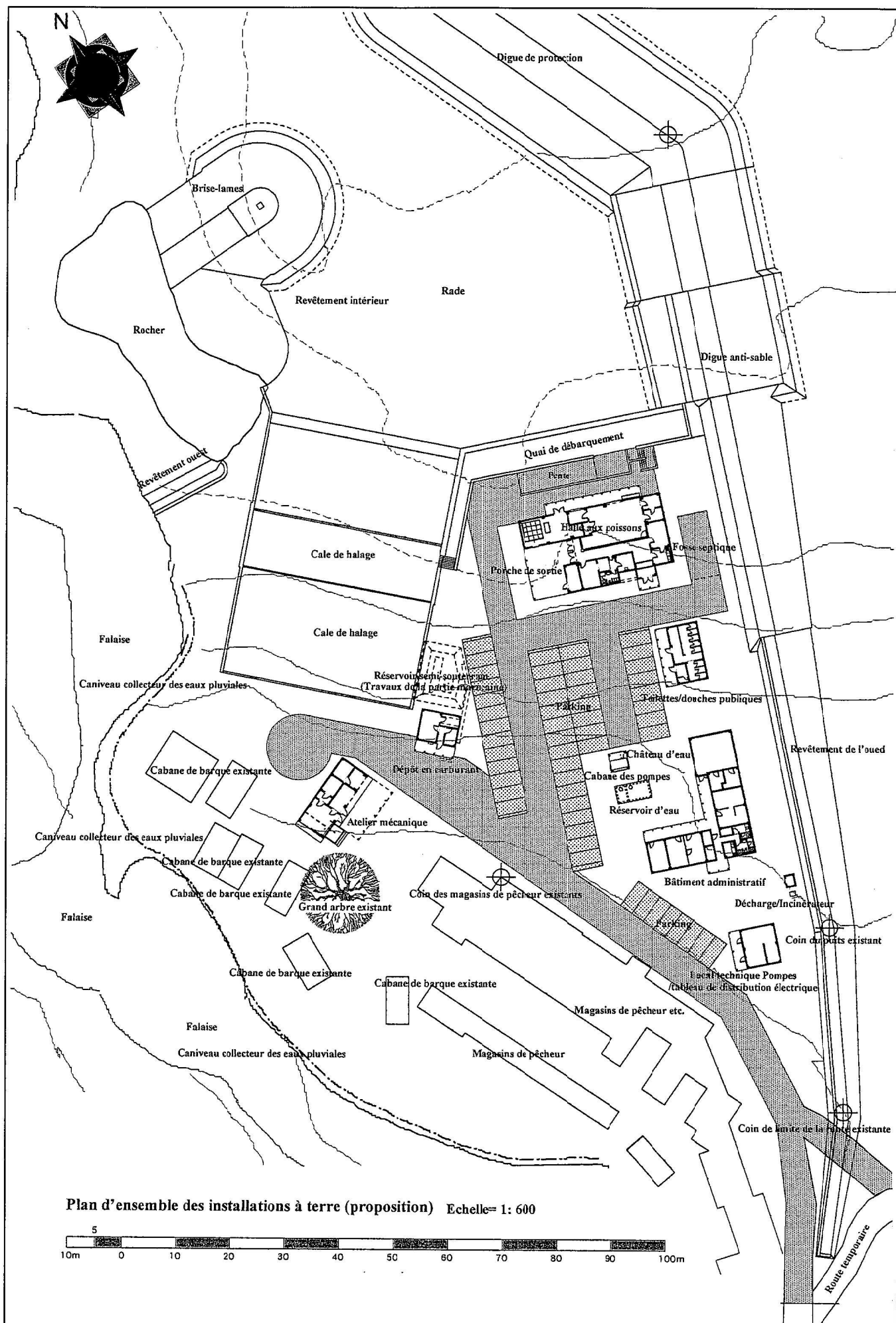
Plan 2.2.4-22 Plan d'ensemble des installations à terre (proposition)
