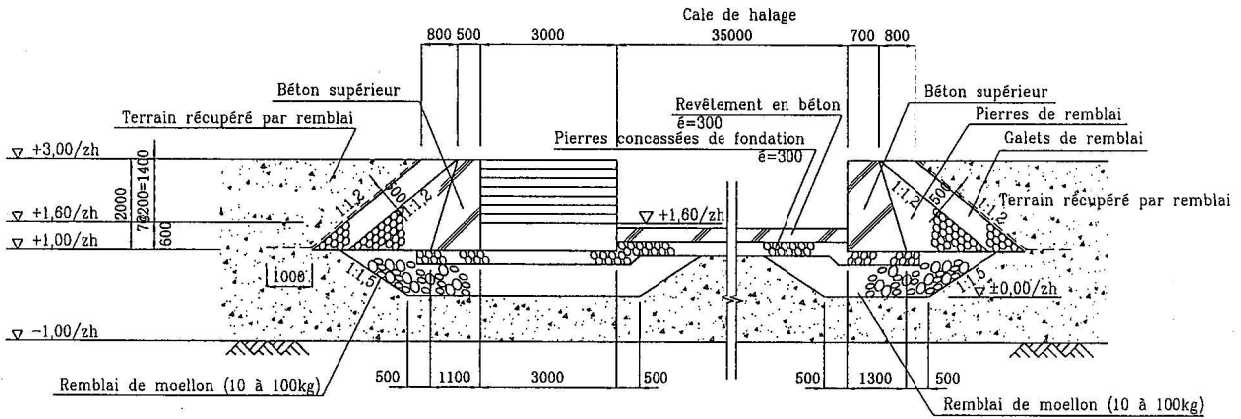
Plan 2.2.4-20 Coupe du mur latéral de la cale de halage (D)
