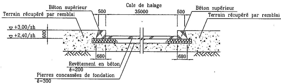
Plan 2.2.4-21 Coupe du mur latéral de la cale de halage (E)
