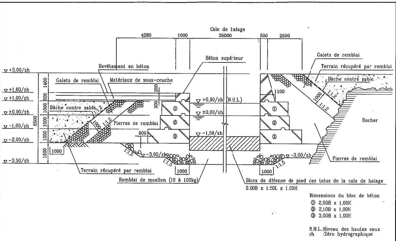
Plan 2.2.4-17 Coupe du mur latéral de la cale de halage (A)
