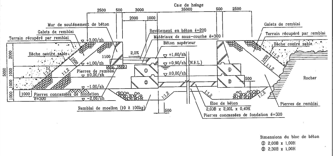
Plan 2.2.4-18 Coupe du mur latéral de la cale de halage (B)
