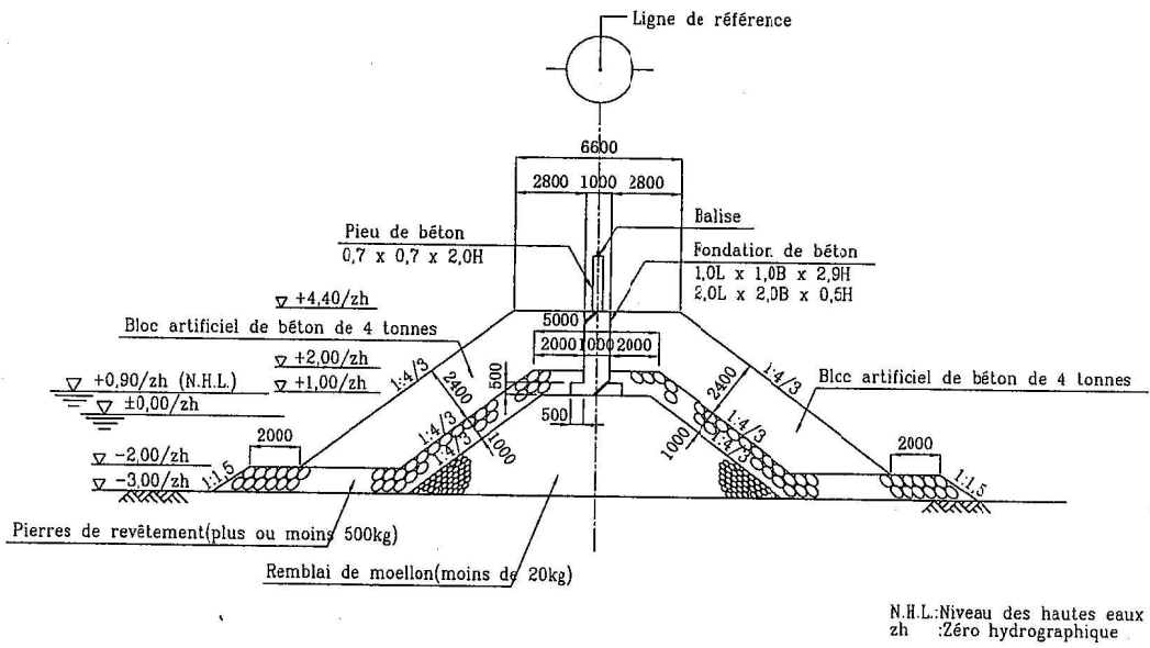
Plan 2.2.4-2 Coupe de la digue de protection (tête de la digue)
