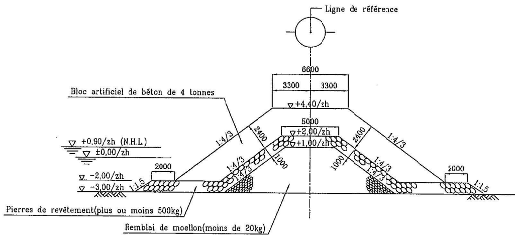
Plan 2.2.4-3 Coupe de la digue de protection (partie du tronc)
