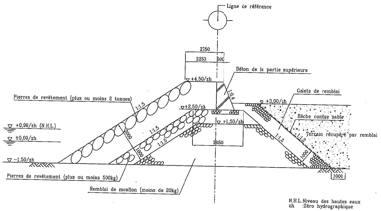
Plan 2.2.4-6 Coupe du revêtement anti-lames
