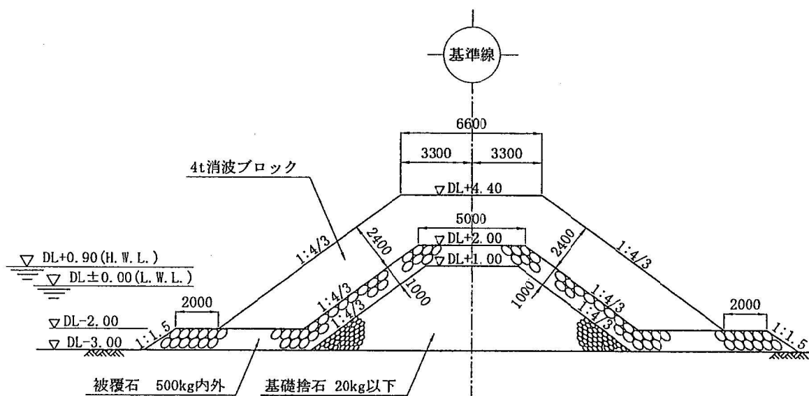
図 3.2.4-3 防波堤堤幹部 断面図
