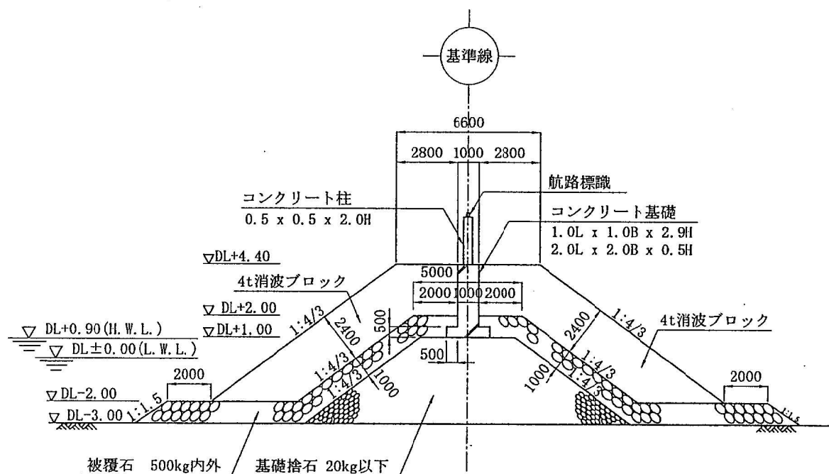
図 3.2.4-2 防波堤堤頭部 断面図
