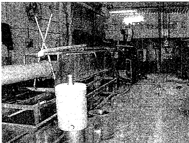
PVCパイプ押し出し成形ライン
