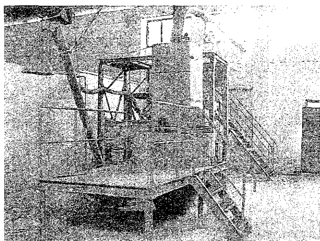
自動供給されるミキサー
