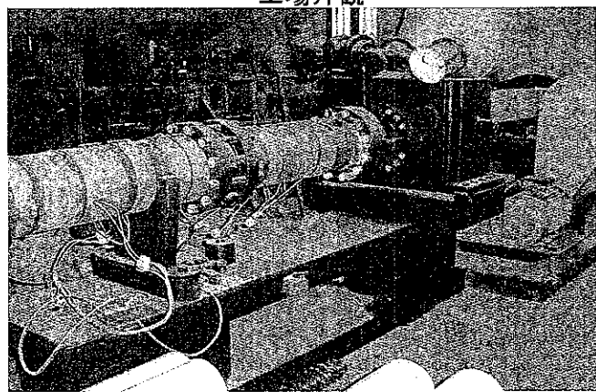
内製のPVCパイプ押出し成形機
