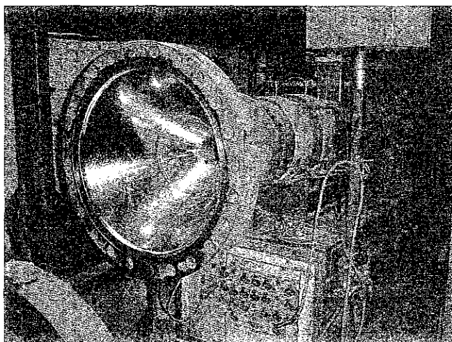
24インチパイプまで可能な内製金型
