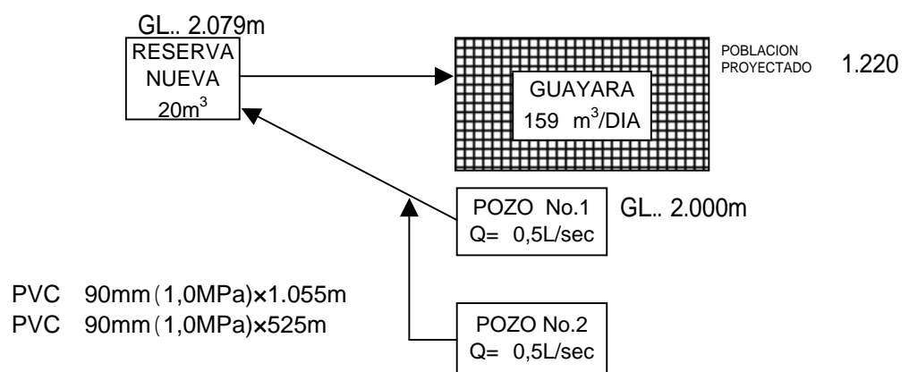
Fig. 2-2-4(8) SISTEMA DE SUMINISTRO DE AGUA No.19 GUAYARA
