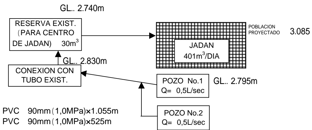
Fig. 2-2-4(5) SISTEMA DE SUMINISTRO DE AGUA No.12 JADAN
